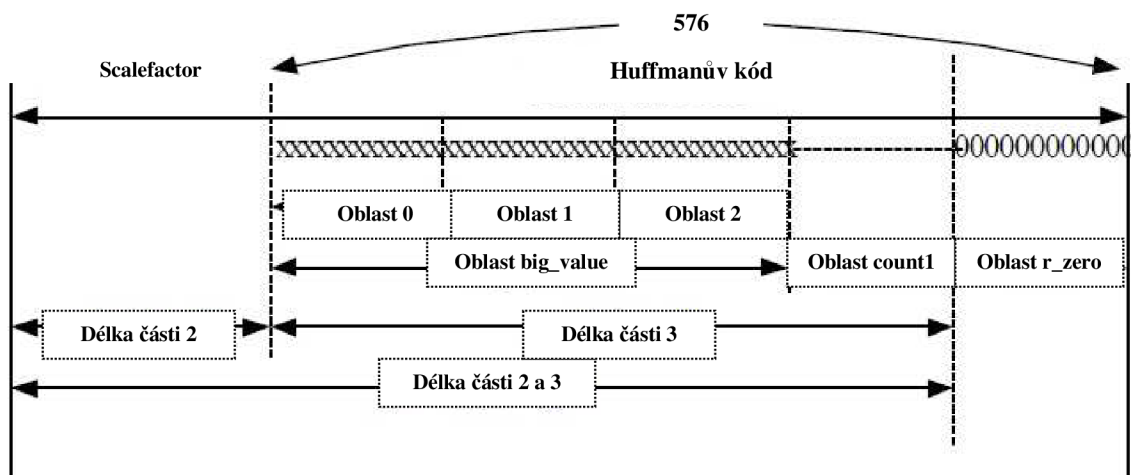
Obrázek 8: Huffmanovo kódování [7]
