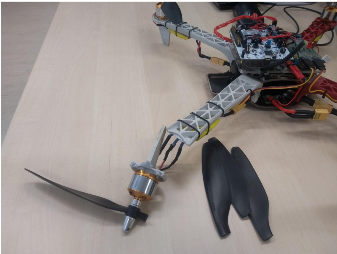
Obr. 73: Poškozená kvadrokoptéra
