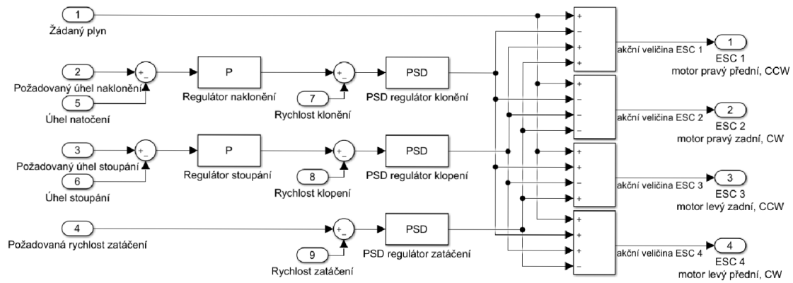
Obr. 7: Regulační obvod
