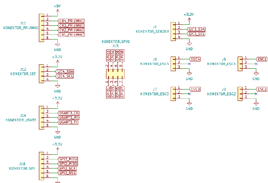
Obr. 46: Zapojení konektorů
