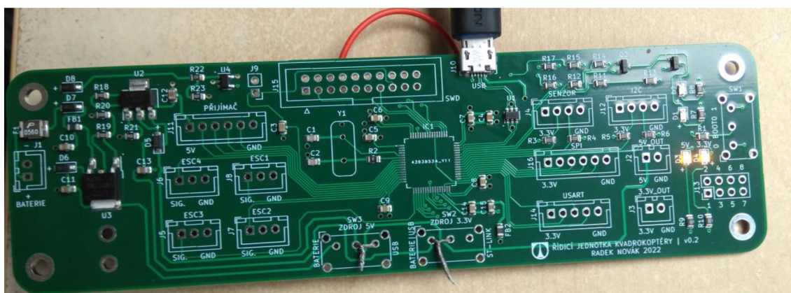
Obr. 60: Vyrobena deska během základního testování
