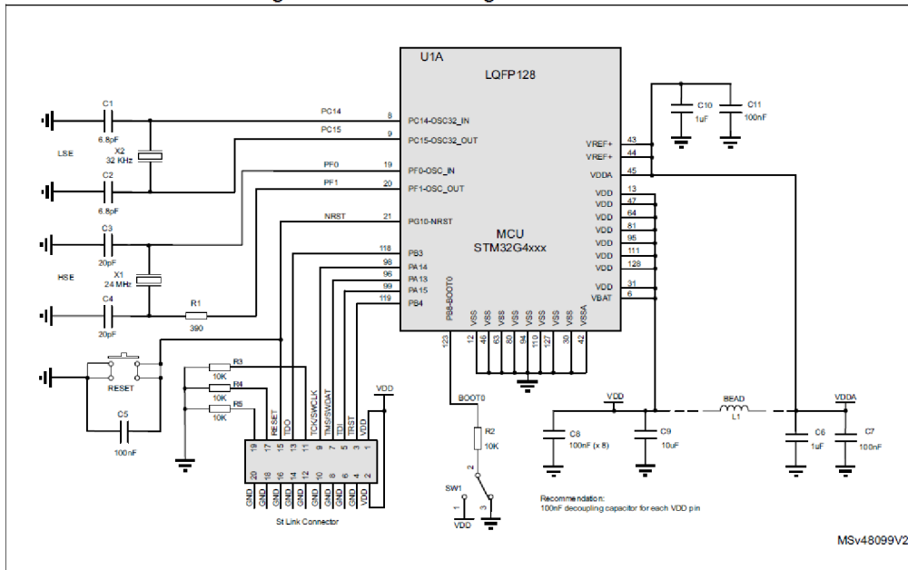
Obr. 39: Referenční schéma zapojení [48]
