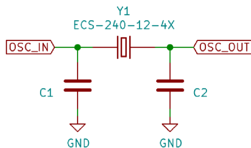
Obr. 44: Zapojení krystalu
