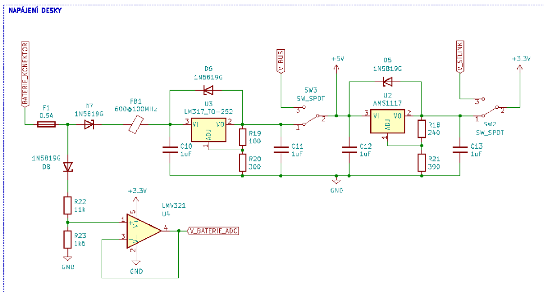
Obr. 37: Blok napájení desky
