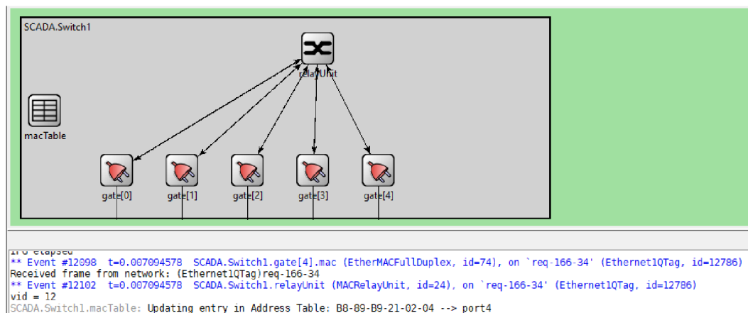
Obr. 3.8: Průběh komunikace v reálném čase v zařízení Switch1
