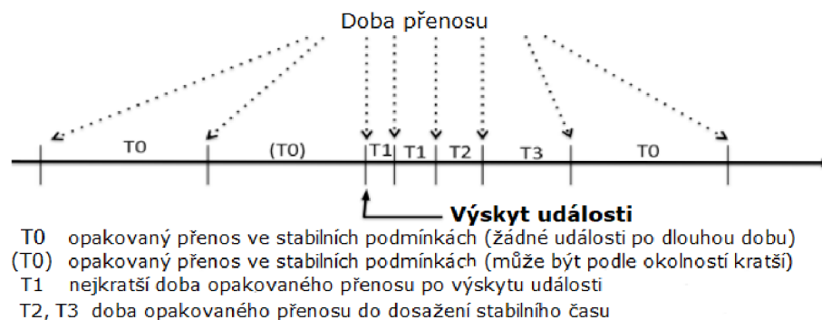
Obr. 1.6: Časový interval přenosu GOOSE zpráv, převzato z [12].
