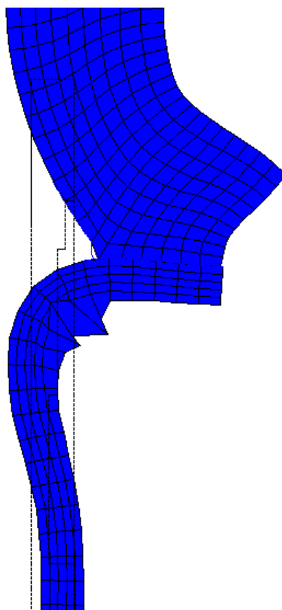
Obr. 7.12: Zborcení sítě
