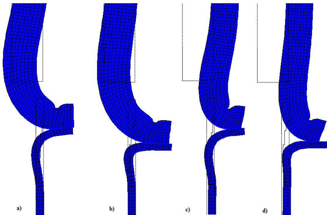
Obr. 7.16: Deformovaný a neděformovaný tvar: a) před zatížením 1. iterace b) před zatížením poslední iterace c) po zatížení vnitřním tlakem 1. Iterace d) po zatížení vnitřním tlakem poslední iterace
