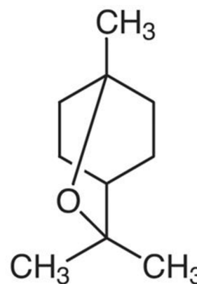
Obr.č.7: 1,8-cineol (1,8-cineole, 2022)
