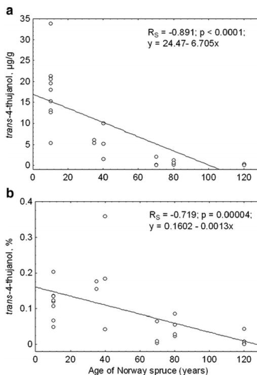
Obr.č.6: Vztah mezi stářím smrku ztepilého a koncentrací ( \mu\text{g/g} sušiny kůry), jakož i relativním množstvím (%), vztaženo na 13 monoterpenu trans -4-thujanolu (Blažytě-Čereškienė, a další, 2016)
