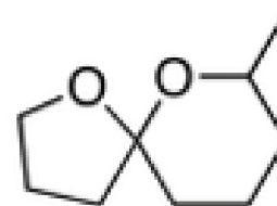
Obr.č.5 Vzorec Trans -konophthorin (Unelius, 2014)
