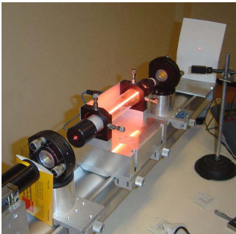
Obr. 1.14 Helium-neonový laser (47)
