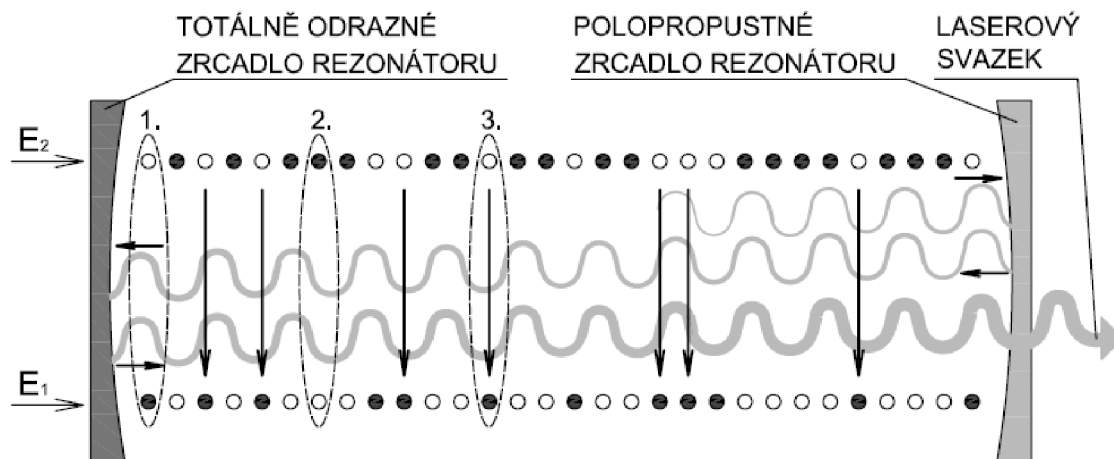
Obr. 1.16 Optický rezonátor (36)
