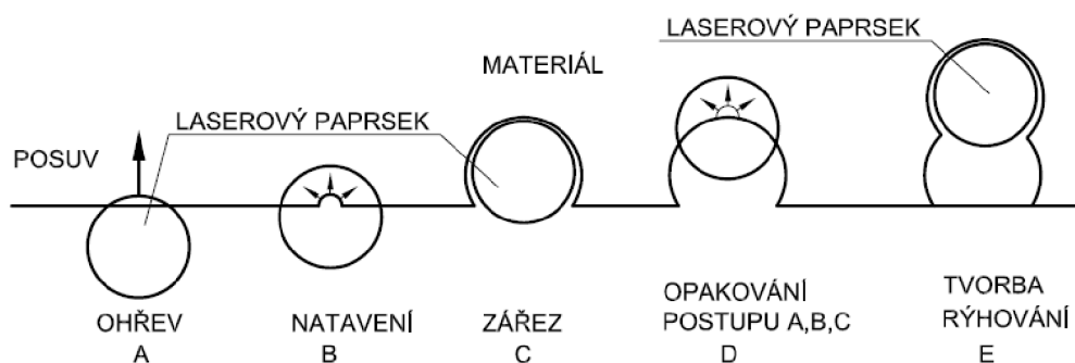
Obr. 1.22 Model tvoření rýh v zóně tavného řezání laserem (22)
