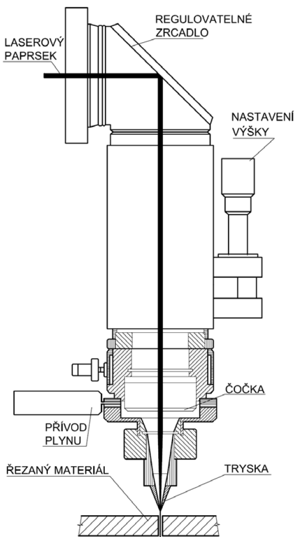
Obr. 1.24 Řezací hlavičce (15)
