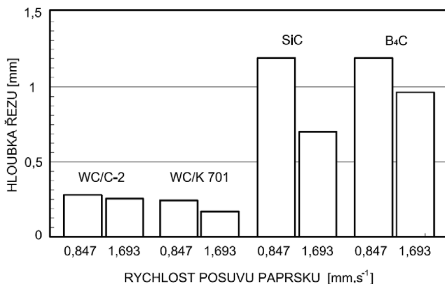
Obr. 2.14 Hloubka řezu pro materiály s odlišnou tvrdostí a houževnatostí (22) Podmínky řezání: d_n=0,457 mm, d_m=1,14 mm, l_m=50 mm, p=311 MPa, m_a=12,7 g.s -1 , brusivo granát zrnitost 80
