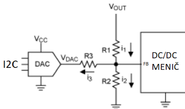
Obrázok 3.1 Zapojenie D/A prevodníku v obvode spätnej väzby, prekreslené z [5]
