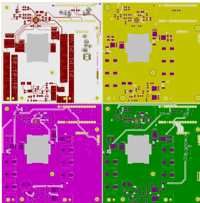
Obrázok 8.1 Prehľad vrstiev navrhovanej DPS, horný rad zľava: prvá (vrchná) a druhá vrstva, dolný rad zľava: tretia a štvrtá (spodná) vrstva
