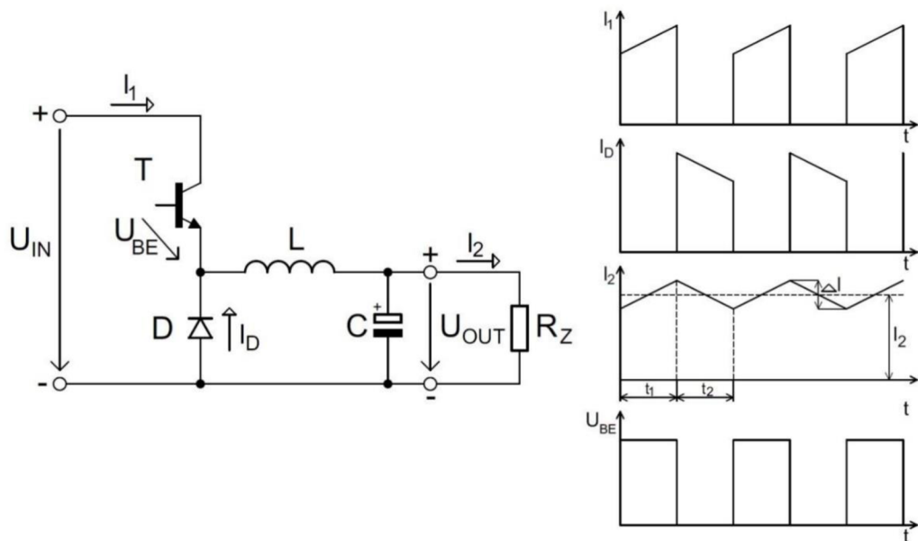
Obrázok 2.2 Schéma znižujúceho meniča a časové priebehy prúdov a napätí v obvode, prevzaté z [3]
