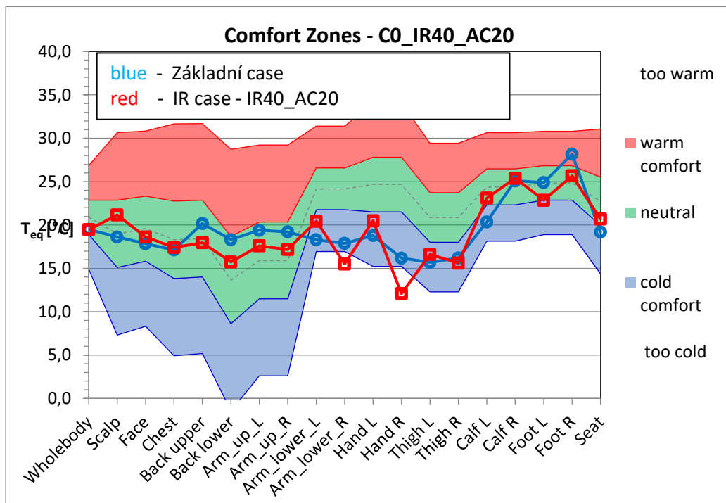
Graf2.20.40: Case T_{amb}=0\text{ °C} T_{IR}=40\text{ °C} T_{AC}=20\text{ °C}
