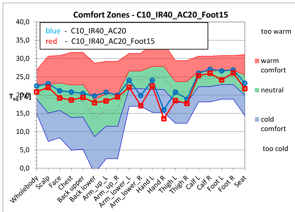
Graf 4.20.40-3: Case T_{amb}=10\text{ }^{\circ}\text{C} T_{IR}=40\text{ }^{\circ}\text{C} T_{Ac}=20\text{ }^{\circ}\text{C} , teplota vzduchu z výustky nižší o 5 °C k základnímu scénáři
