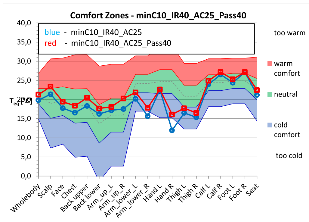
Graf 6.25.40-2: Case T_{amb} = -10\text{ °C} T_{IR} = 40\text{ °C} T_{AC} = 25\text{ °C} , teplota panelů dveří a střeby pasažéra T = 40\text{ °C}
