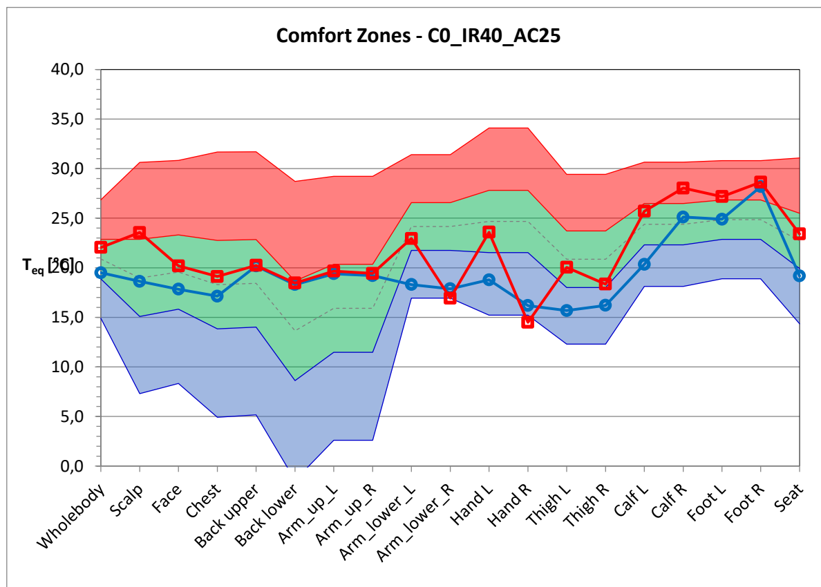
Graf 3: Komfortní zóny scénáře 2.25.40
