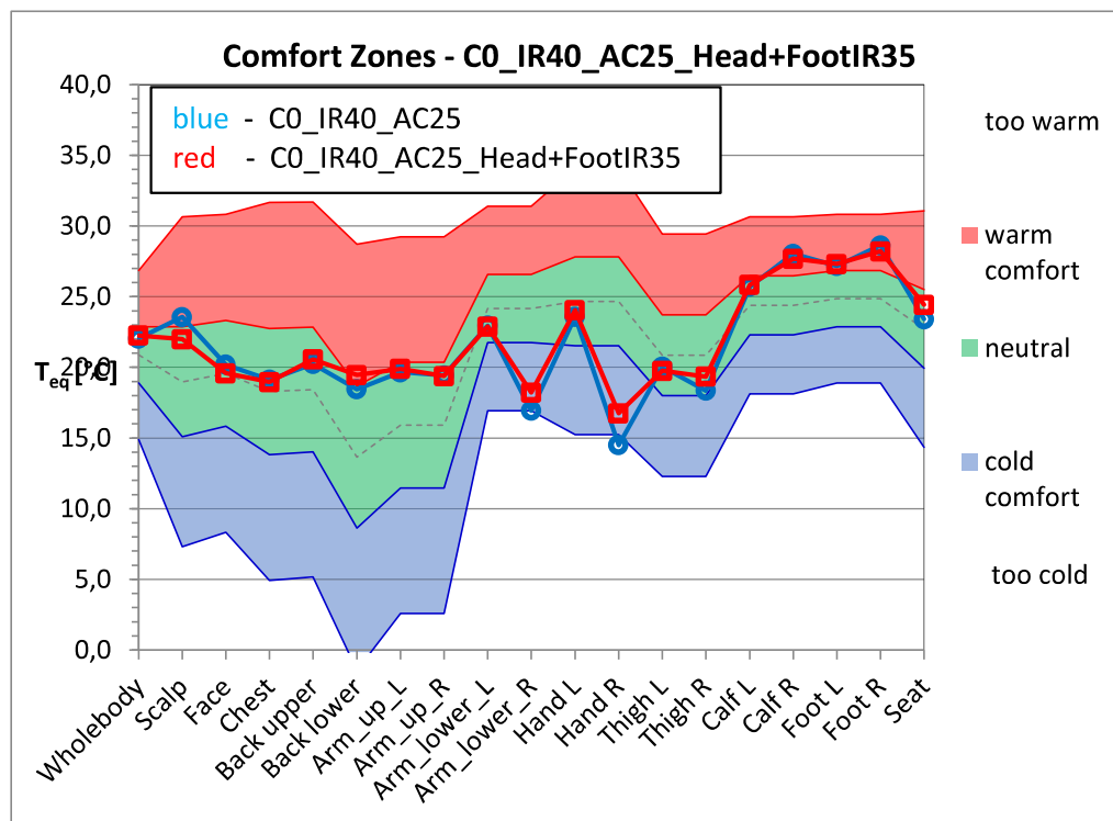
Graf 5.25.40-1: Case T_{amb}=0\text{ °C} T_{IR}=40\text{ °C} T_{AC}=25\text{ °C} , teplota panelů dveří a střechy T=35\text{ °C}
