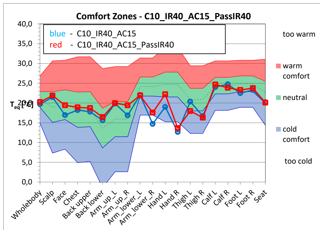
Graf 4.15.40-2: Case T_{amb}=10\text{ }^{\circ}\text{C} T_{IR}=40\text{ }^{\circ}\text{C} T_{AC}=15\text{ }^{\circ}\text{C} , teplota panelů dveří a střežy pasažéra T=40\text{ }^{\circ}\text{C}
