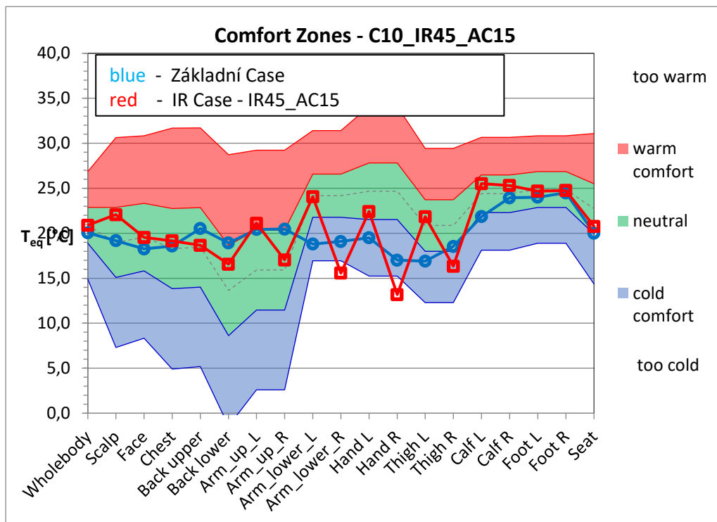
Graf 1.15.45: Case T_{amb}=10\text{ °C} T_{IR}=45\text{ °C} T_{AC}=15\text{ °C}
