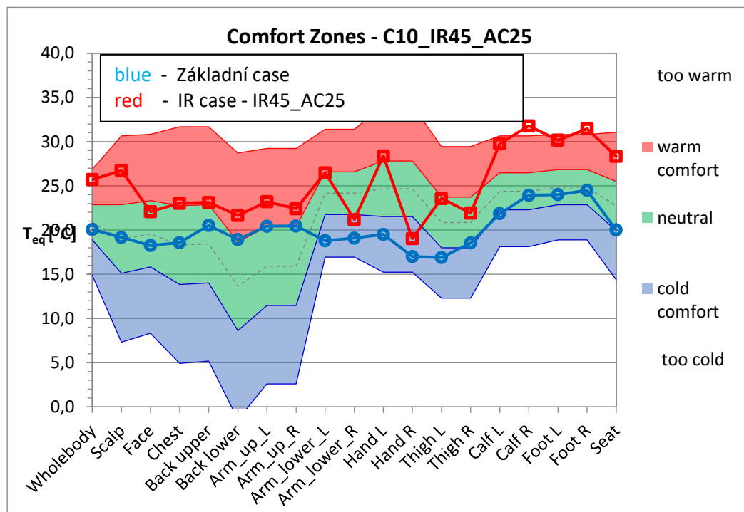
Graf 1.25.45: Case T_{amb}=10\text{ }^{\circ}\text{C} T_{IR}=45\text{ }^{\circ}\text{C} T_{AC}=25\text{ }^{\circ}\text{C}
