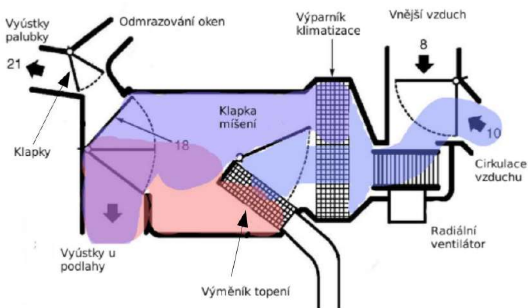
Obrázek 2: Schéma vedení vzduchu systémem HVAC [1]
