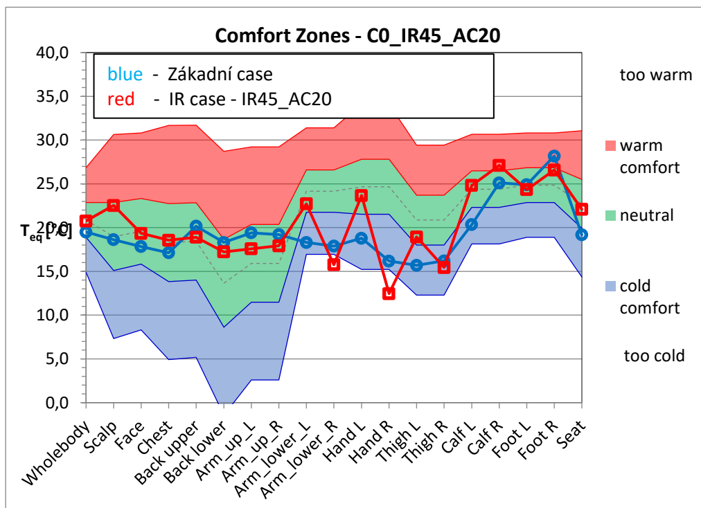
Graf2.20.45: Case T_{amb}=0\text{ °C} T_{IR}=45\text{ °C} T_{AC}=20\text{ °C}
