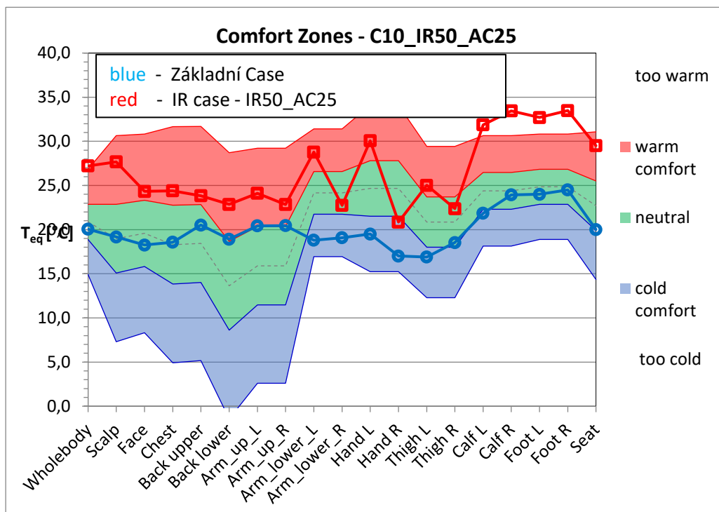
Graf 1.25.50: Case T_{amb}=10\text{ }^{\circ}\text{C} T_{IR}=50\text{ }^{\circ}\text{C} T_{AC}=25\text{ }^{\circ}\text{C}
