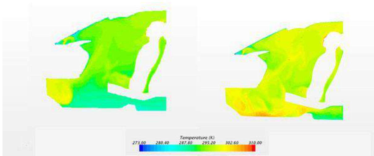
Obrázek 14: Porovnání vlivu směřování proudu z vyústky pro nohy - 0^\circ (obrázek vlevo) a 30^\circ k normále plochy (obrázek vpravo)
