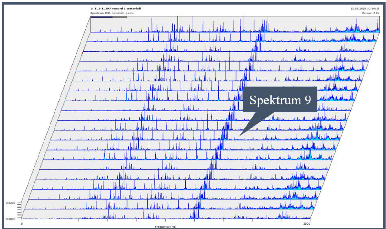
Obr. 19) Vodopádový graf osy x (1. meranie, čelné obrábanie, SKF)
