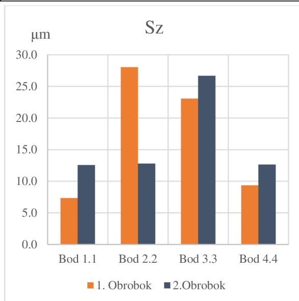
Obr. 18) Histogram zobrazujúci porovnanie parametra Sz
