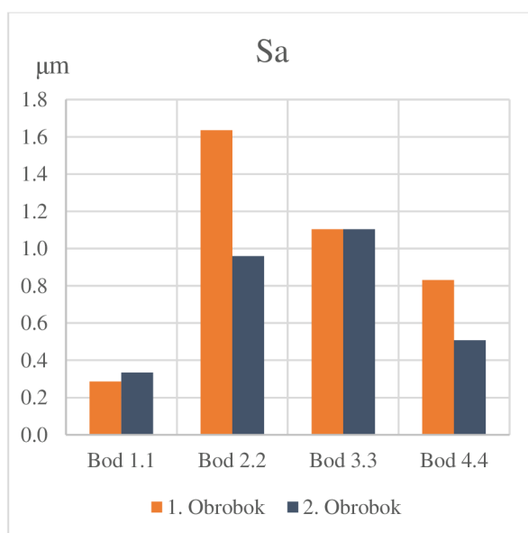
Obr. 19) Histogram zobrazujúci porovnanie parametra Sa
