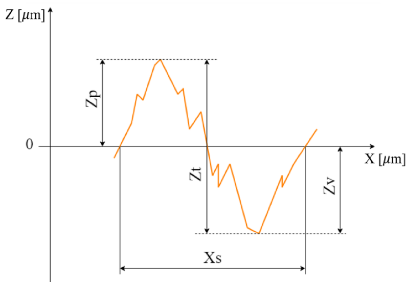
Obr. 15) Prvok profilu
