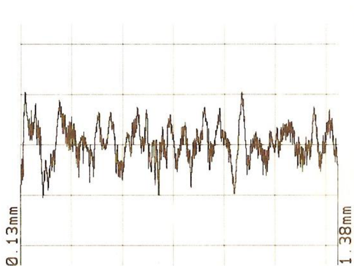
Obr. 2.4 Dosahované parametry střední aritmetické úchylky profilu R_a 0,145 .
