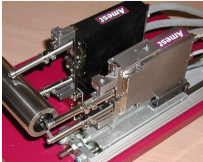
Obr. 4.12 Sledovací měřidlo vnějšího a vnitřního průměru Amest [3].
