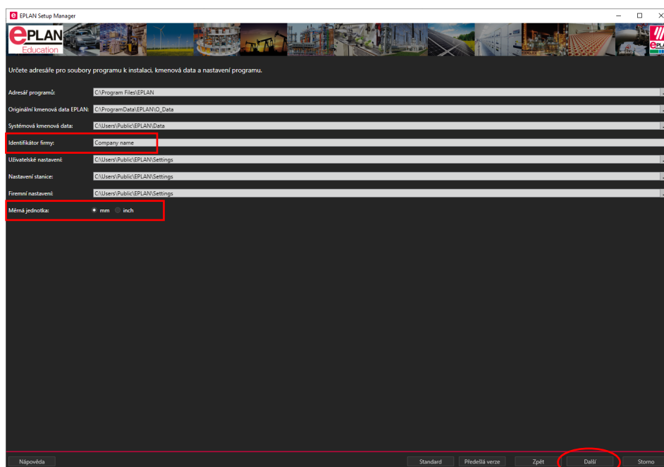
Obrázek 3.7 Nastavení adresářů
