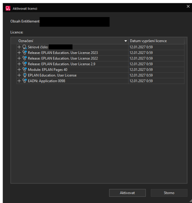
Obrázek 3.11 Obsah licence
