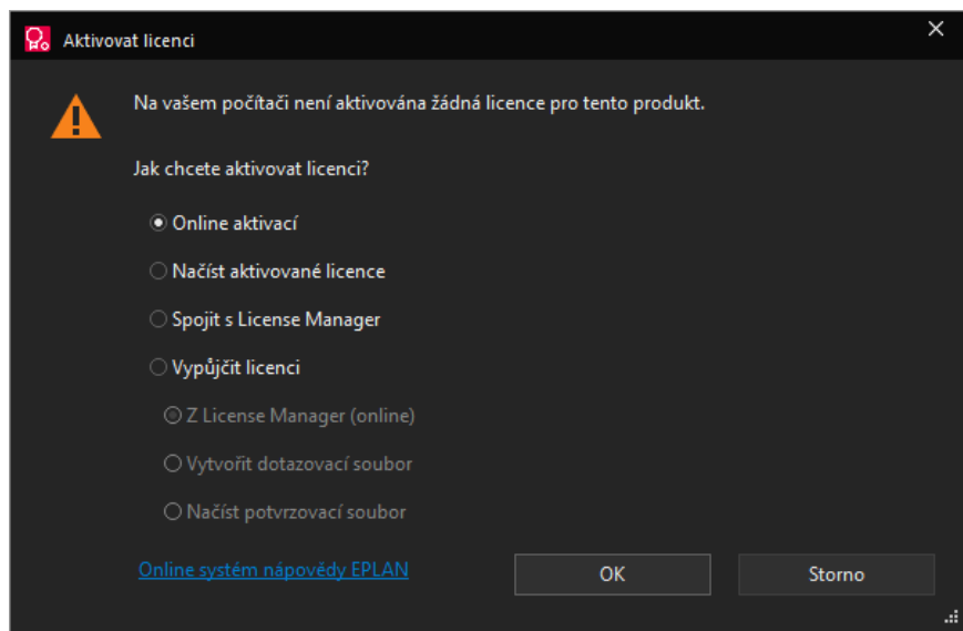
Obrázek 3.9 Aktivace licence
