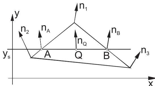
Obrázok 5.6: Lineárna interpolácia normálových vektorov
