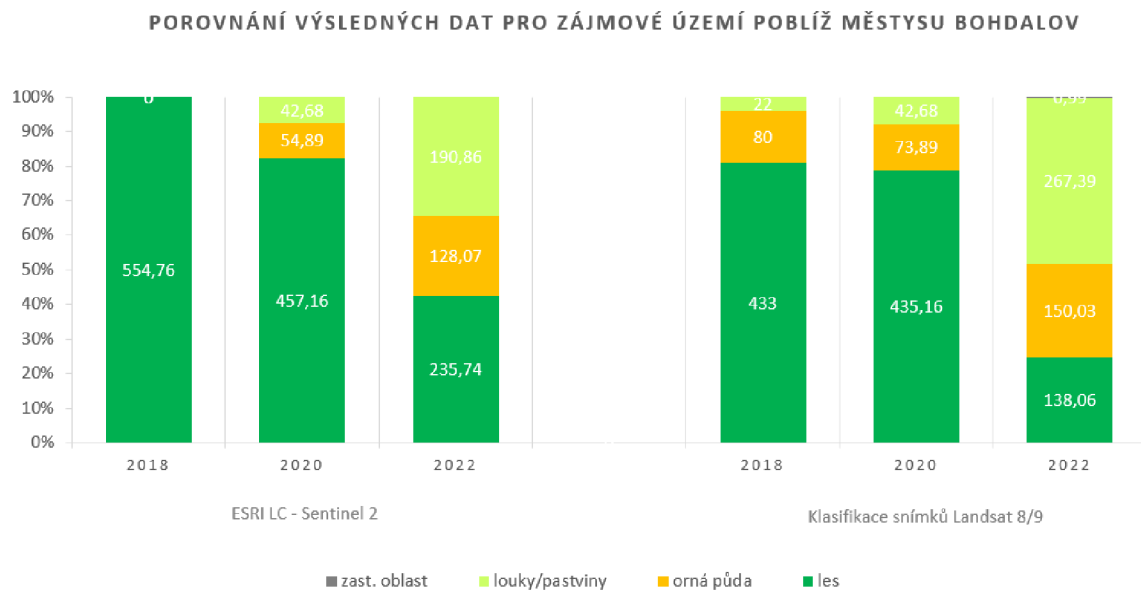
Graf 1: Grafické znázornění krajinného pokryvu pro zájmové území poblíž městyso Bohdalov
