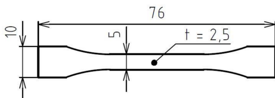
obr. 4-3 rozměry tělesa 1BA pro tahovou zkoušku
