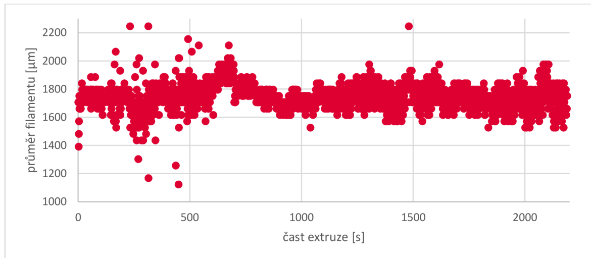
obr. 6-1 průměry filamentu v průběhu extruze při prvním recyklačním cyklu
