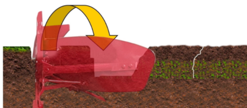
Obr. 14 – Radlice pluhu (zdroj: Charrues Demblon)
