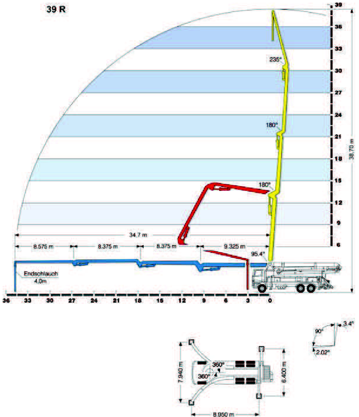
Obr.A.3.7 Dosah autočerpáda
