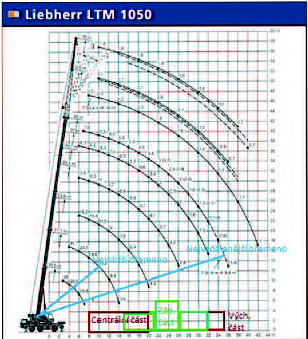
Obr.A.3.11 Dosah autojeřábu včetně zakreslení budovy stacionáře.
