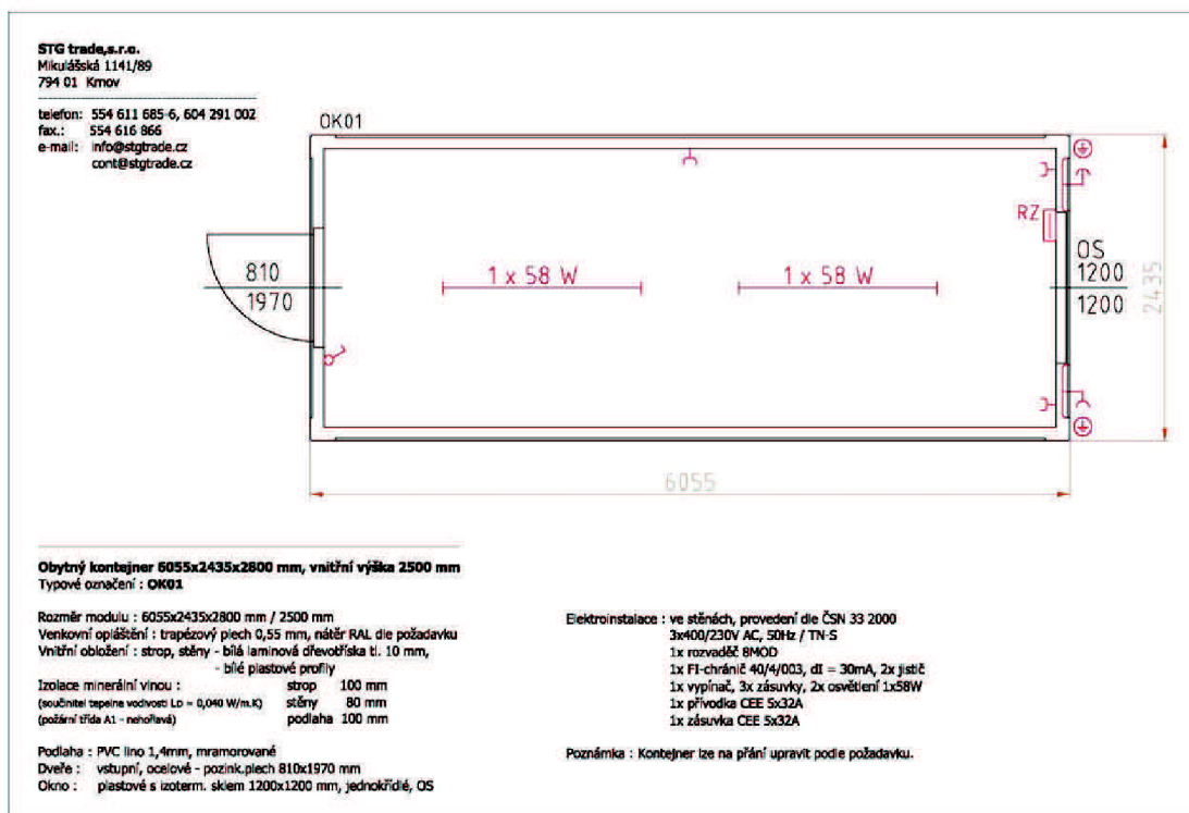
Obr. A.4.2 Půdorys obytného kontejneru OB 01
