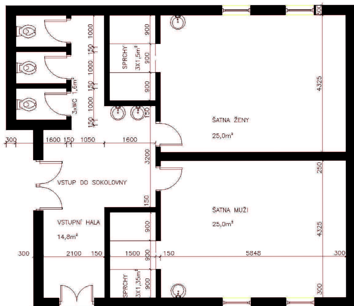
Obr. A.4.1 Půdorys sociálního zařízení pro pracovníky umístěného v sokolovně
