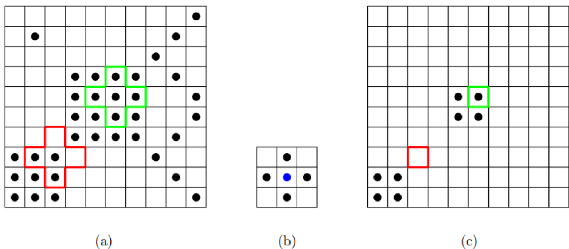
Obr. 3.1: Schématické znázornění binární eroze. (a) vstupní binární obraz, tečkami jsou znázorněny jedničky binárního obrazu, zeleně je ohraničena aktivní poloha strukturálního elementu, červeně je ohraničena neaktivní poloha strukturálního elementu. (b) Strukturální element s vyznačeným centrálním referenčním prvkem. (c) Výstupní obraz binární eroze, prvek v červeném rámečku byl odstraněn, prvek v zeleném rámečku byl zachován [29]
