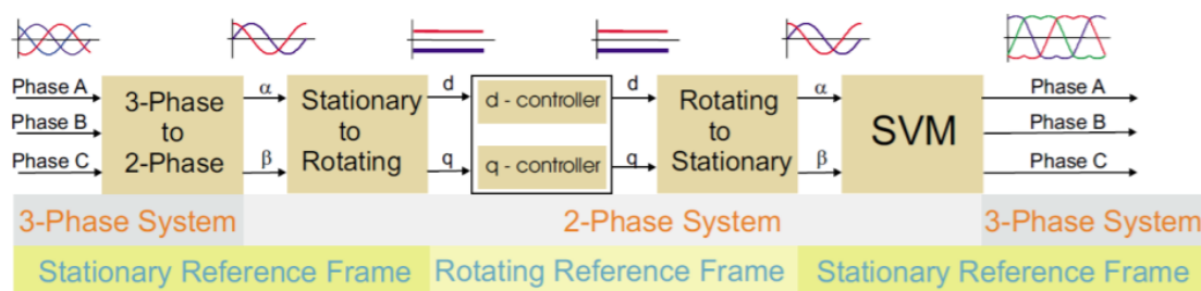
Obrázek 6.1 - Transformace signálů ve vektorovém řízení [12]
