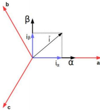
Obrázek 5.1 - Clarkové transformace [10]
