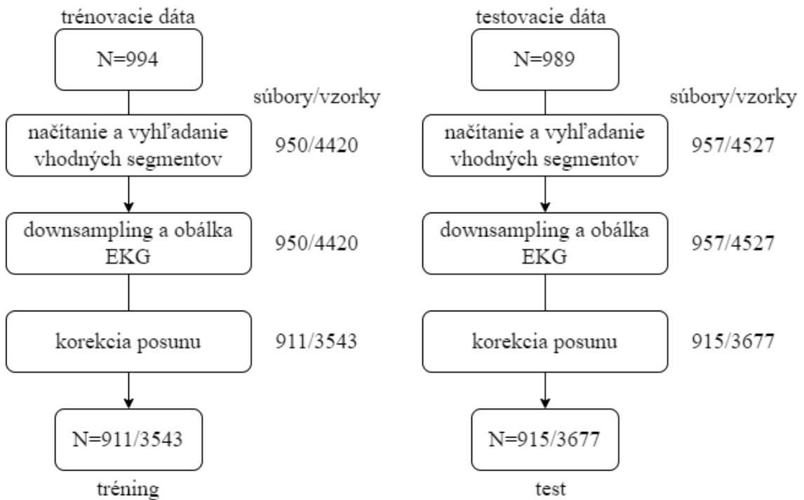
Obr. 4.6: Schéma úbytku dát v dôsledku ich spracovania. Trénovacie a testovacie dáta rešpektujú pôvodné rozdelenie zo serveru PhysioNet. Trénovacia sada bola použitá pre vývoj modelu (tréning a validácia), testovacia pre záverečný test.
