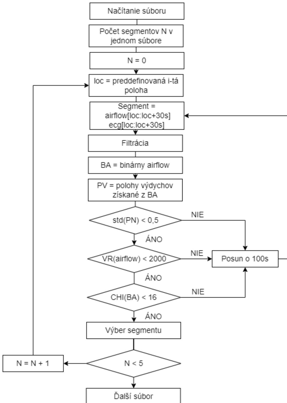
Obr. 4.2: Schéma postupu získania dát z jedného súboru.
