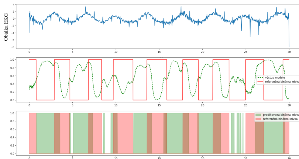
Obr. 4.14: Ukážka zlého odhadu binárnej respiračnej krivky, IOU=0,2. Chybná činnosť algoritmu je pravdepodobne spôsobená poškodením EKG signálu, ktorý neobsahuje validné dáta a poukazuje na nedokonalosť algoritmu pre výber segmentov.
