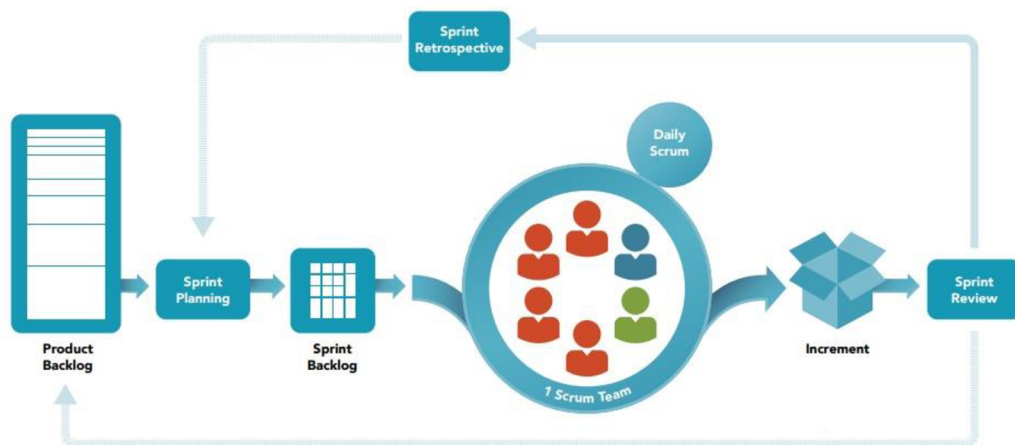
Obrázek 7 - SCRUM proces [19]
