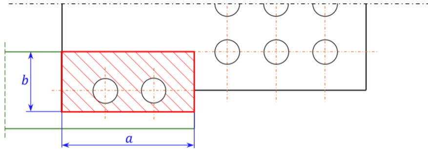
Obrázek 5.14 Kontaktní styková plocha mezi praporec a spojovací destičkou
