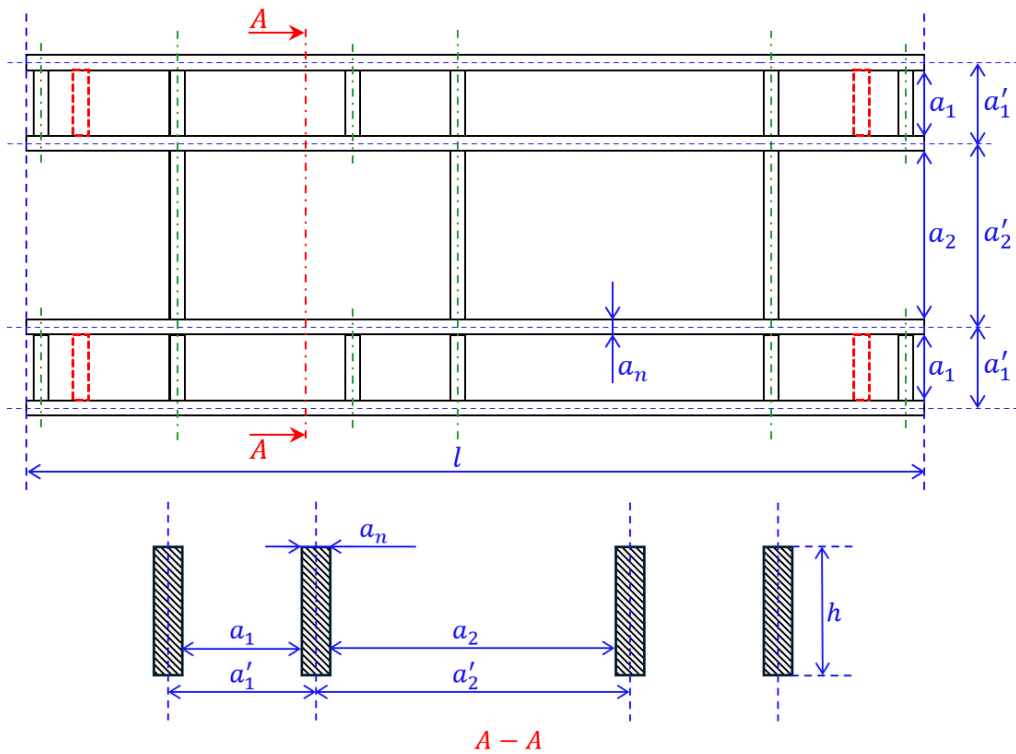
Obrázek 5.3 Soustava nožů jedné fáze
