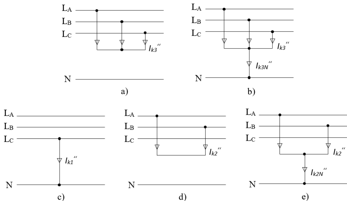
Obrázek 2.3 Druhy zkratů [8]:
