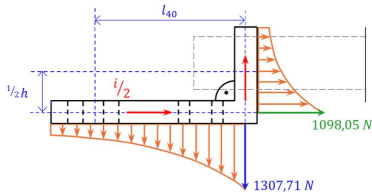
Obrázek 5.8 Rozložení vypočtených sil na pravoúhlý záhyb praporce
