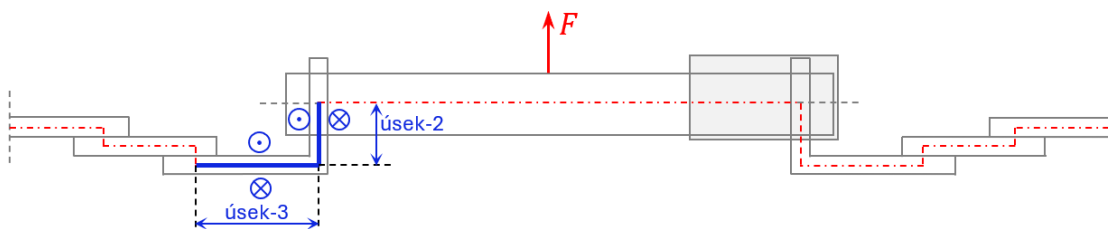
Obrázek 5.5 Úseky 2 a 3 proudovodné dráhy odpojovače KBE
