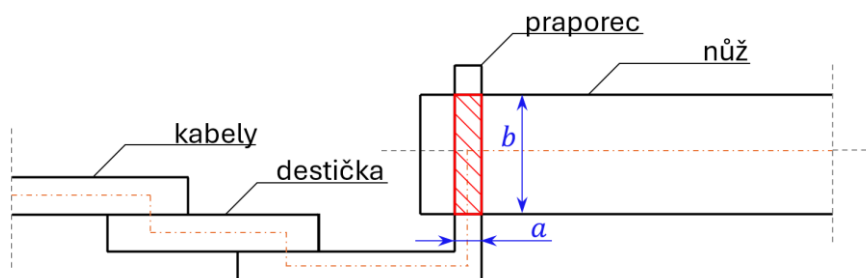
Obrázek 5.12 Kontaktní styková plocha mezi praporecem a nožem
