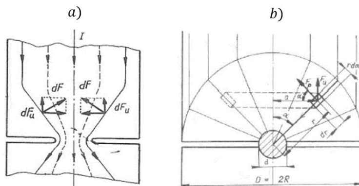
Obrázek 5.11 Odpuvivé síly v proudové úžině (a) a idealizované proudové úžině (b) [9]
