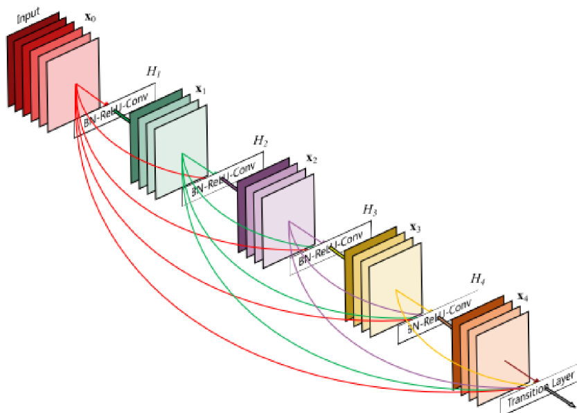
Obrázek 39: Znárodnění Densenet, Zdroj: https://amaarora.github.io/images/densenet.png
