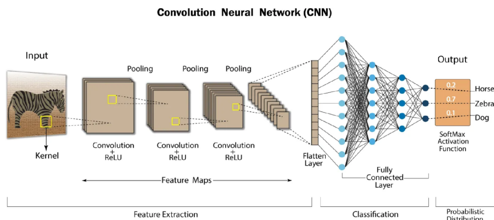
Obrázek 2: Diagram konvoluční sítě, Zdroj: https://i0.wp.com/developersbreach.com/wp-content/uploads/2020/08/cnn_banner.png?fit=1400%2C658&ssl=1
