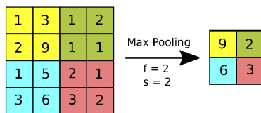
Obrázek 4: Diagram pooling vrstvy, Zdroj: https://anhreynolds.com/blogs/cnn.html
