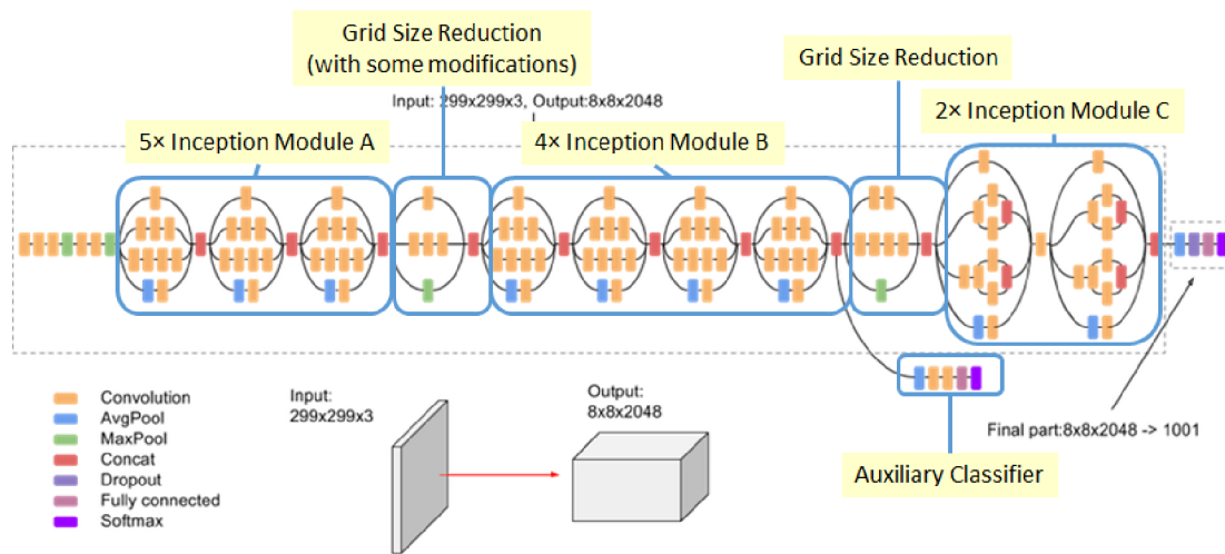
Obrázek 31: Architektura InceptionV3, Zdroj: https://cdn-images-1.medium.com/max/1200/1*gqKM5V-uo2sMFFPDS84yJw.png
