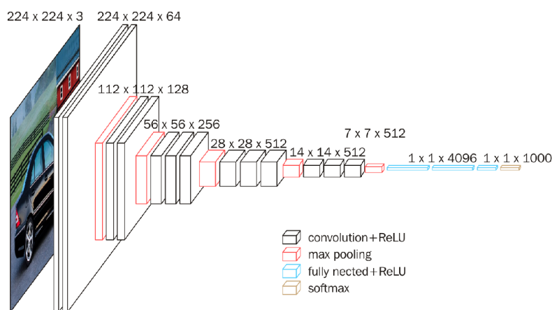
Obrázek 21: Architektura VGG16, Zdroj: https://cdn-images-1.medium.com/max/1600/1* A_uro4dKSBUPWfng8jrPug.png
