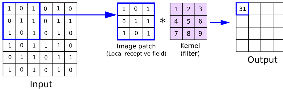
Obrázek 3: Diagram konvoluční vrstvy, Zdroj: https://anhreynolds.com/blogs/cnn.html
