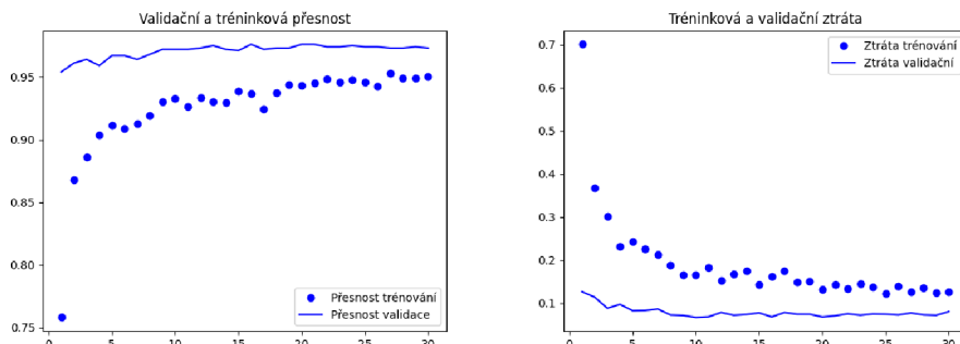
Obrázek 41: Výsledky Densenet121 extr. příz. s rozšířením, Zdroj: Vlastní
