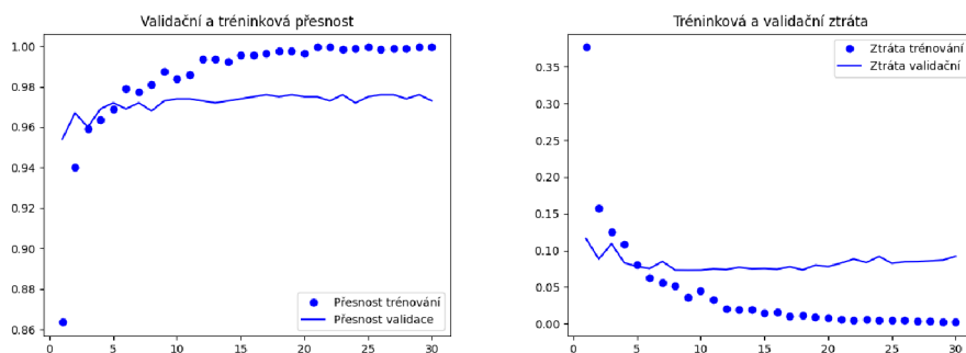
Obrázek 40: Výsledky Densenet121 extrakce příznaků, Zdroj: Vlastní
