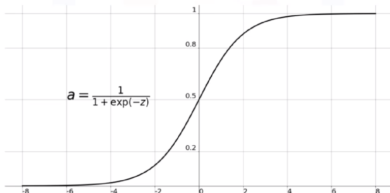
Obrázek 7: Znázornění funkce Sigmoid, Zdroj: https://miro.medium.com/max/2400/1*a04iKNbchayCAJ7-0QlesA.png
