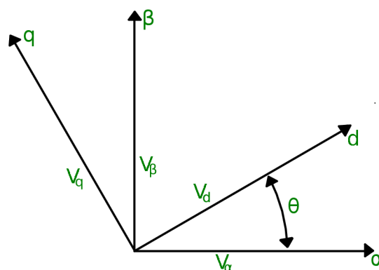
Obr. 1.4: Inverzná Parkova transformácia
