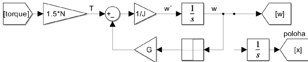
Obr. 7.1: Štruktúra s využitím trenia
