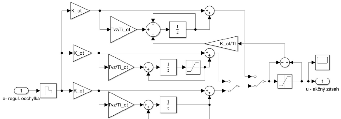
Obr. 4.4: Vnútroštruktúra otáčkového regulátoru \omega
