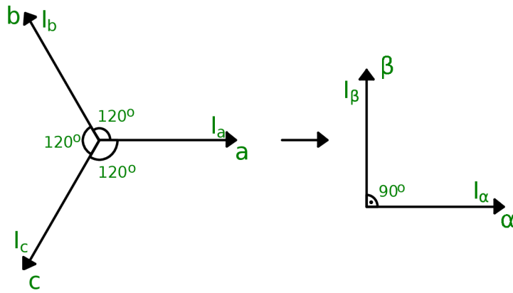
Obr. 1.1: Clarkovej transformácia
