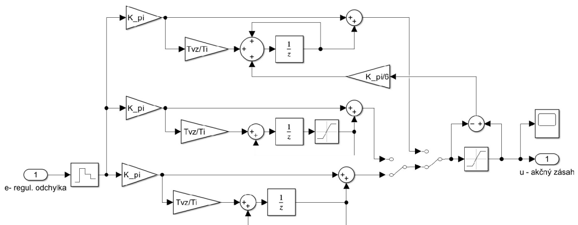
Obr. 4.3: Vnútroštruktúra prúdových regulátorov i_q, i_d
