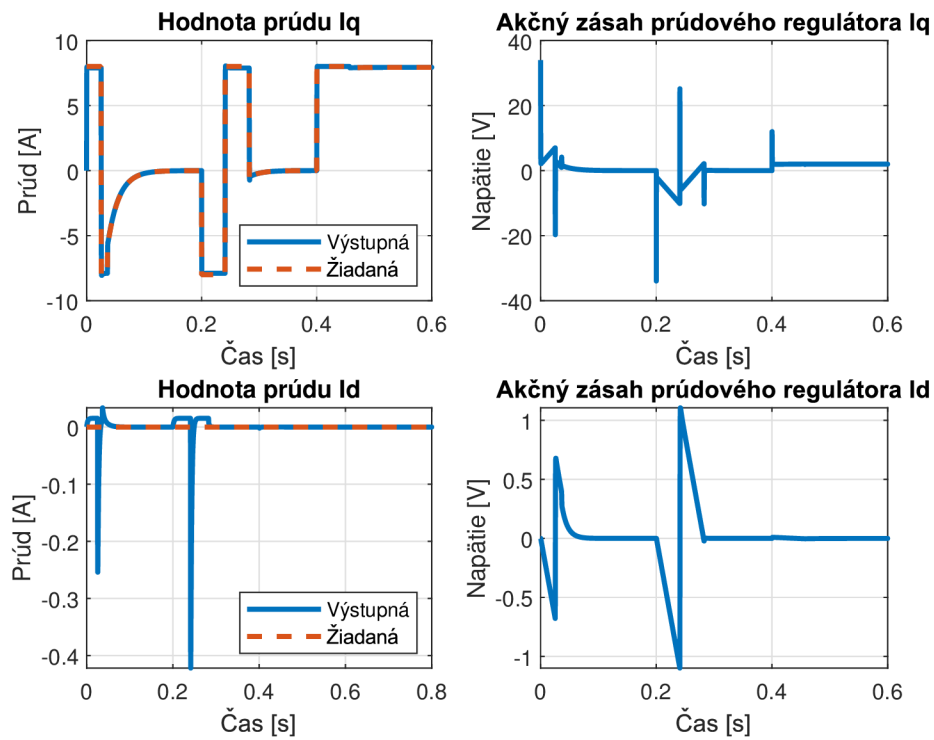
Obr. 4.9: Regulácia na polohu so vstupujúcou poruchou(prúdové regulátory)
