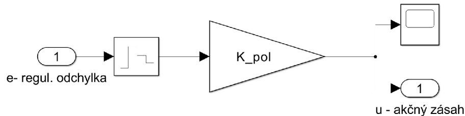
Obr. 4.5: Vnútorná štruktúra polohového regulátoru
