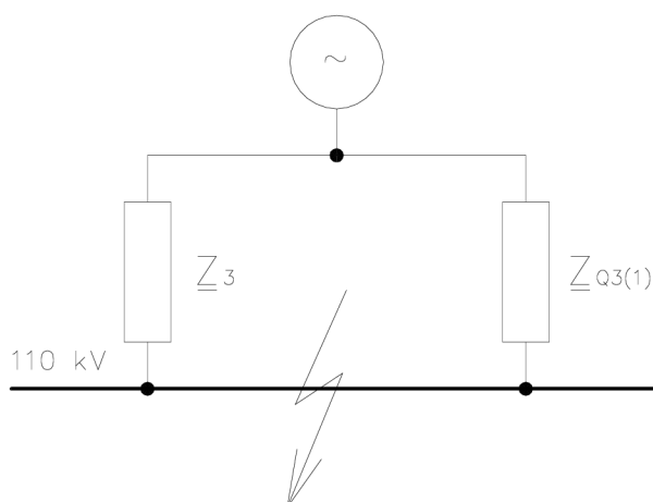
Obr. 3-14 Sériově-paralelní součet impedancí na impedanci \underline{Z}_3
