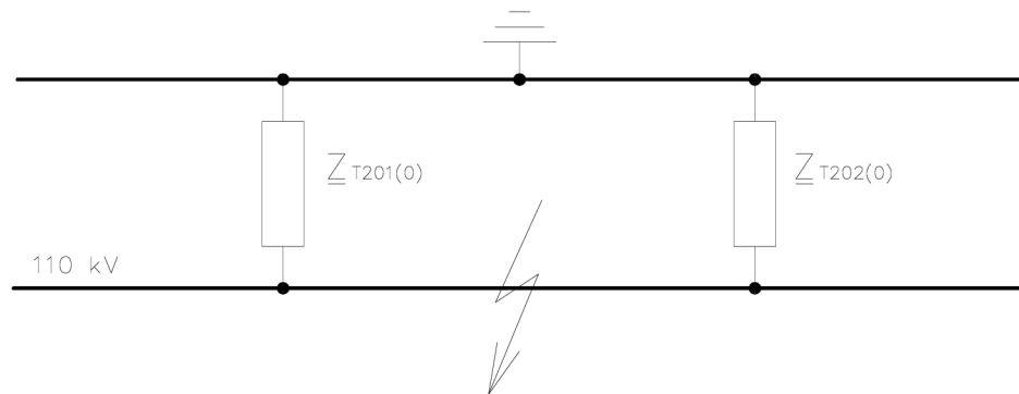
Obr. 3- 18 Celkové impedance transformátorů T201 a T202
