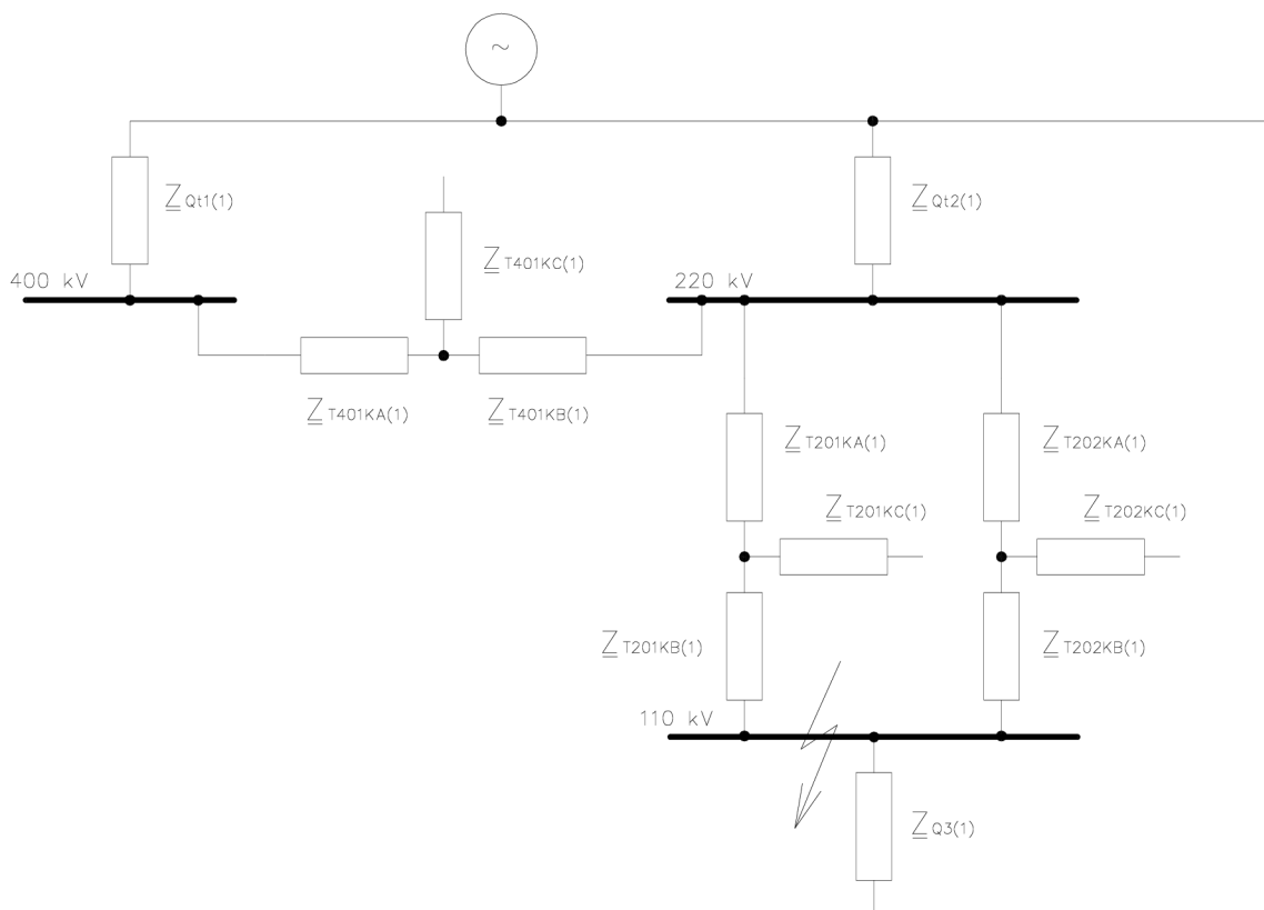
Obr. 3-3 Celý obvod nahrazen souslednými impedancemi
