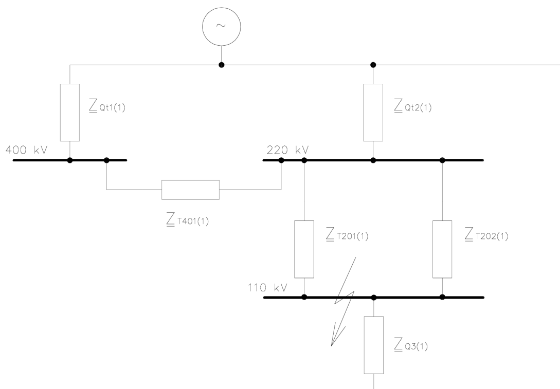
Obr. 3-4 Transformátory nahrazeny jedinou impedancí
