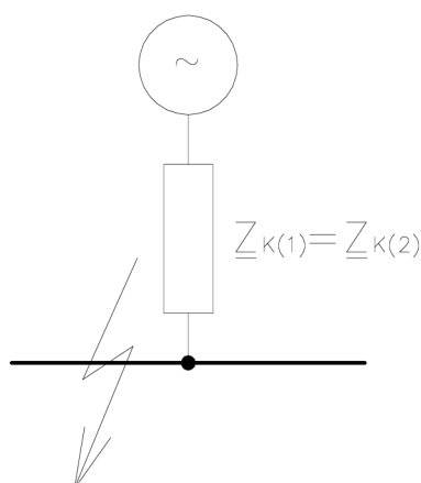
Obr. 3-15 Výsledná zkratová impedance \underline{Z}_{K(1)}
