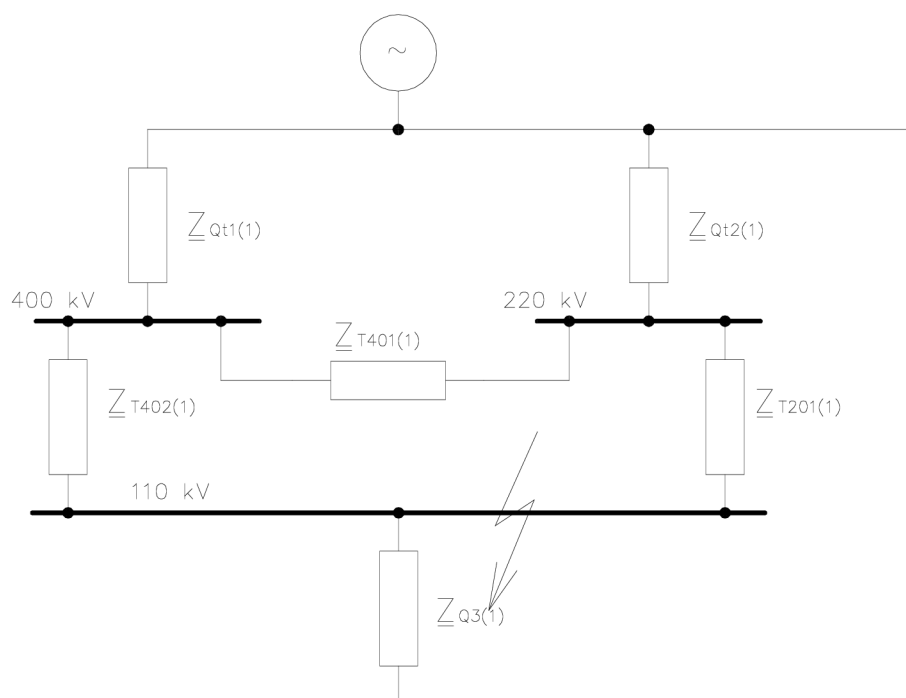
Obr. 3-10 Transformátory nahrazeny jedinou impedancí
