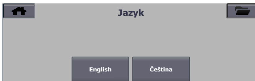
Obrázek 52 – Obrazovka jazyků
