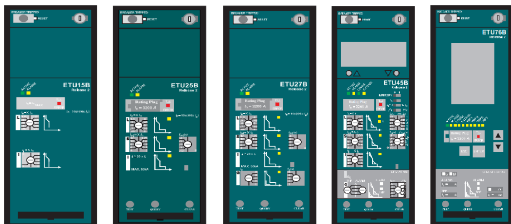
Obrázek 15 – ETU15B, 25B, 27B, 45B, 76B, převzato z [18]
