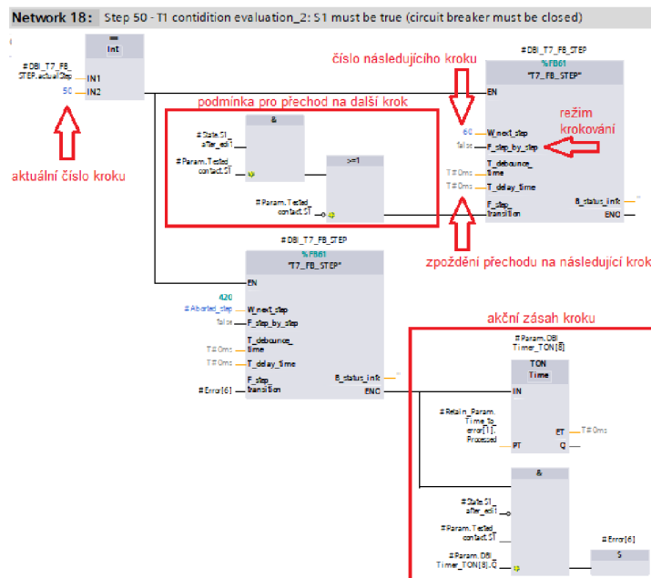
Obrázek 40 – Krok sekvencery
