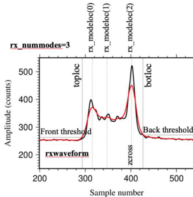
Obrázek č. 4 – Příklad GEDI rxwaveform před (černě) a po (červeně) konvoluci s Gaussovou funkcí šířky 6,5 ns. Algoritmus prohledává pouze část rxwaveform mezi signal_start a signal_end pro odražené mody. Nastavení prahu definuje „nejvyšší“ (nejvíce vlevo, toploc) a „nejnižší“ (nejvíce vpravo, botloc). V tomto příkladu byly algoritmem detekovány tři odlišné mody (rx_nummodes=3). (Hofton et al., 2019)
