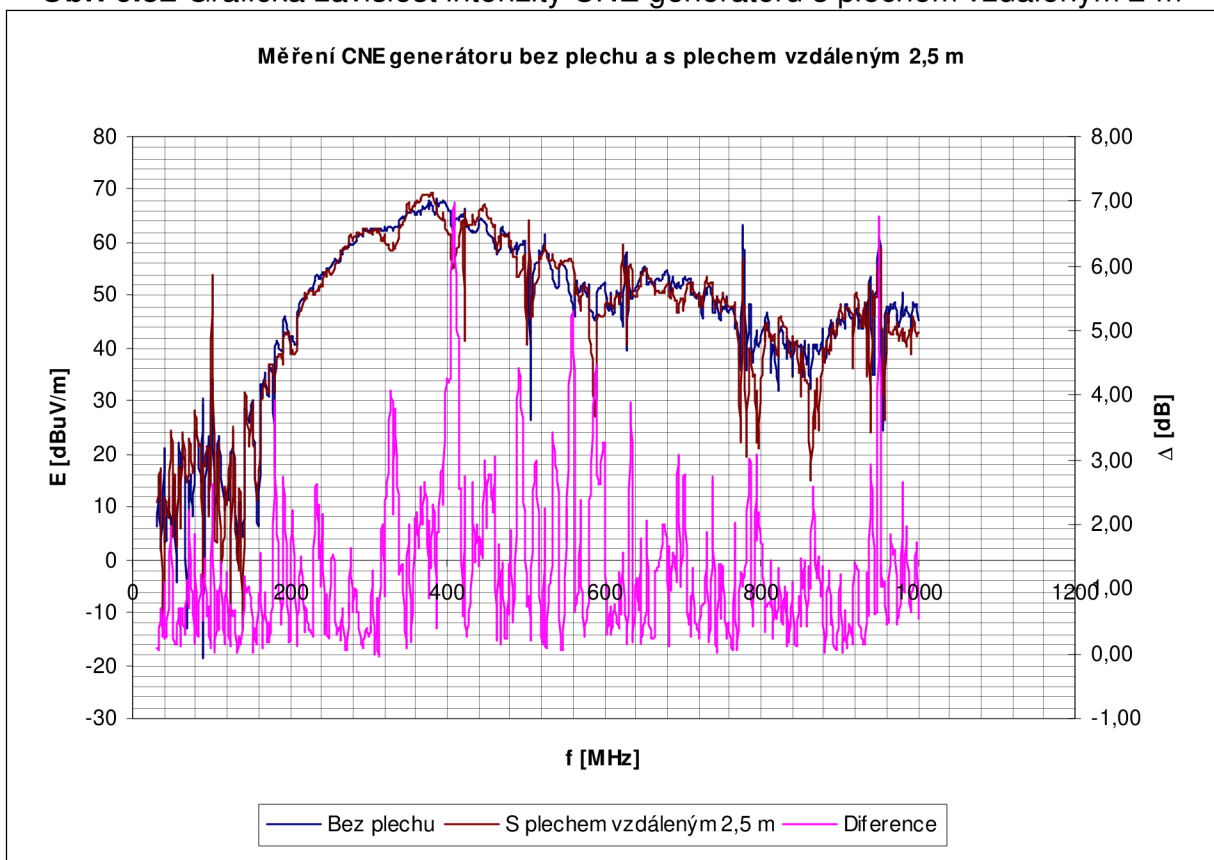
Obr. 6.33 Grafická závislost intenzity CNE generátoru s plechem vzdáleným 2,5 m
