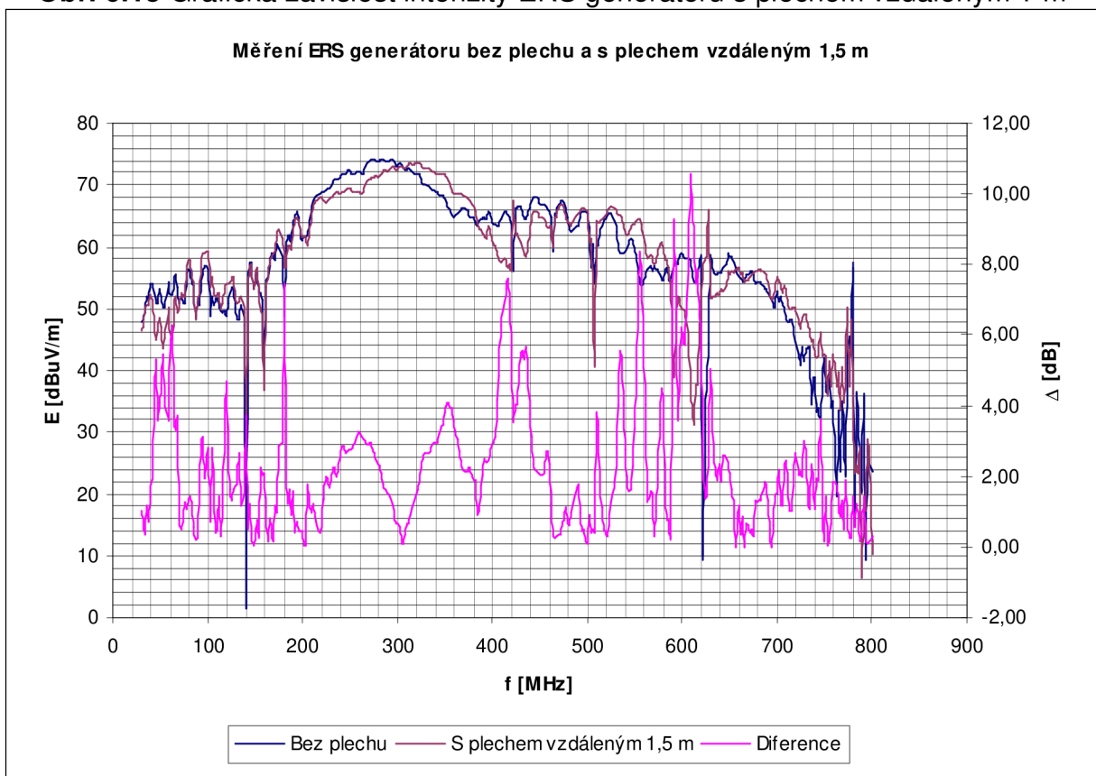
Obr. 6.16 Grafická závislost intenzity ERS generátoru s plechem vzdáleným 1,5 m
