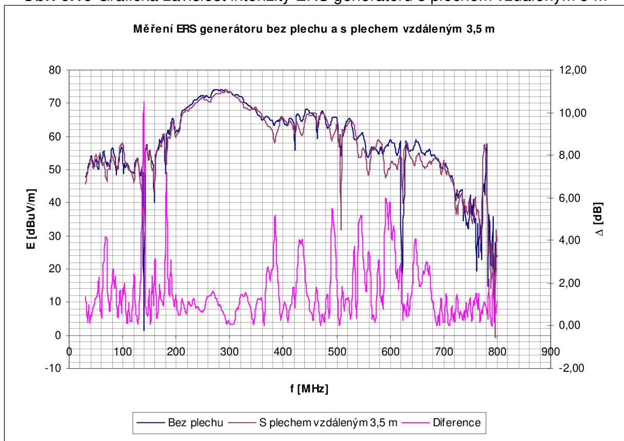
Obr. 6.20 Grafická závislost intenzity ERS generátoru s plechem vzdáleným 3,5 m
