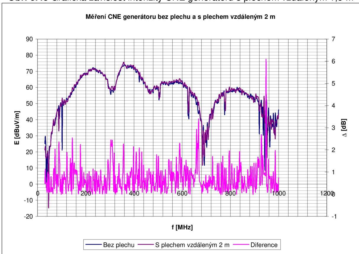
Obr. 6.46 Grafická závislost intenzity CNE generátoru s plechem vzdáleným 2 m
