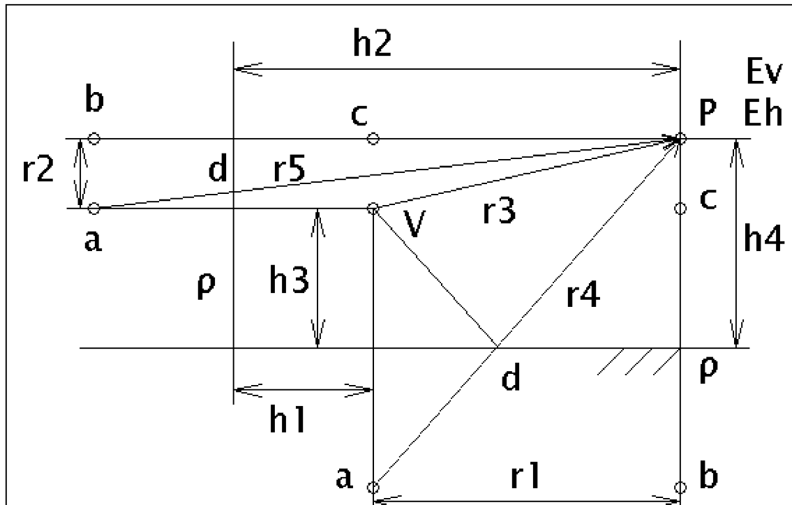
Obr. 5.16 Zobrazení přímé, odražené a odražené vlny od roviny za generátorem
