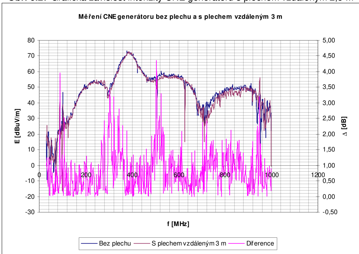
Obr. 6.28 Grafická závislost intenzity CNE generátoru s plechem vzdáleným 3 m
