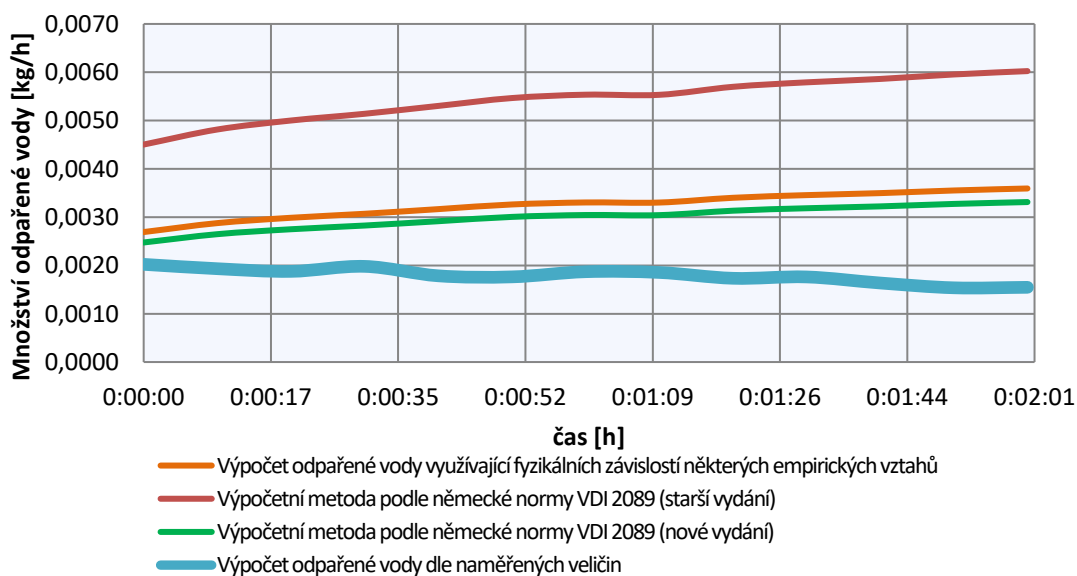
Graf C. 1 – Množství odpařené vody měřením porovnané s některými dalšími výpočtovými metodami pro M1
