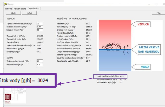
Obr.B. 8 – Výpočet odparu z vířivky
