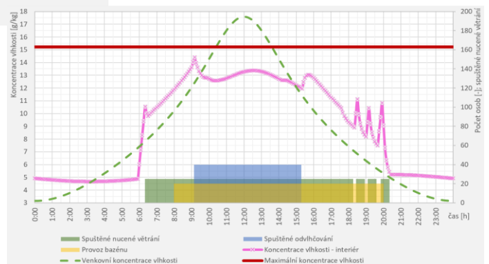
Graf B. 14 – Průběh vlhkosti během dne pro 10/h
