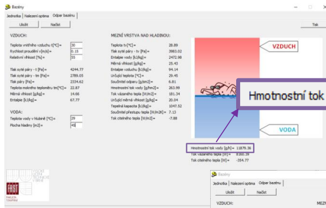
Obr.B. 7 – Výpočet odparu z bazénu
