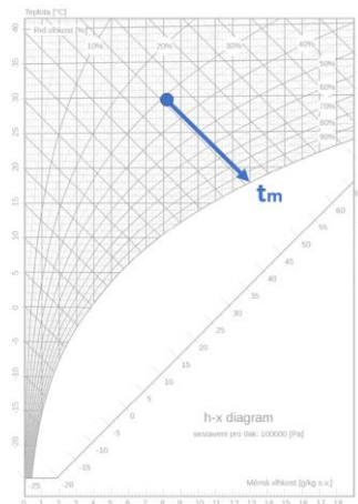
Obr.A. 5 – Teplota mokrého teploměru v h-x diagramu
