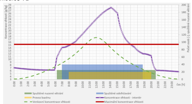
Graf B. 16 - Průběh vlhkosti během dne pro pozici chladiče V2
