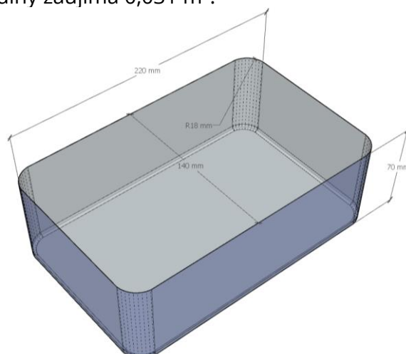
Obr.C. 3 – Geometrie modelu bazény
