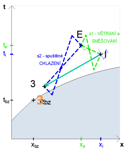
Obr.B. 13 – h-x diagram znázorňující úpravy vzduchu ve V2
