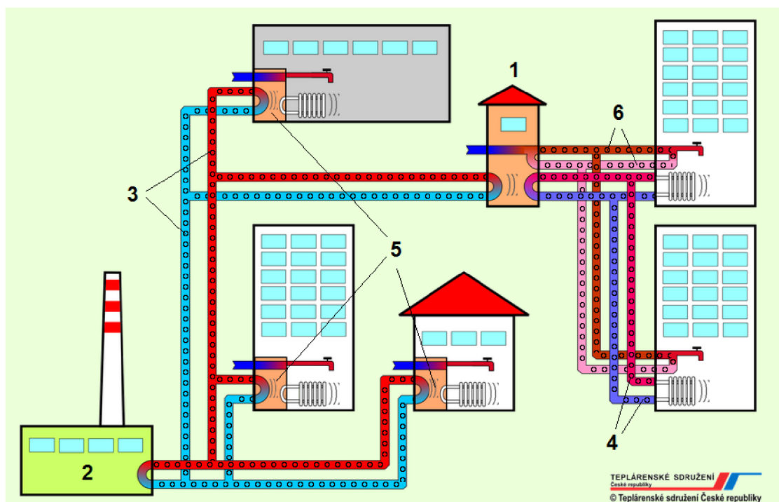
Obr. 3 Soustava CZT [24].
