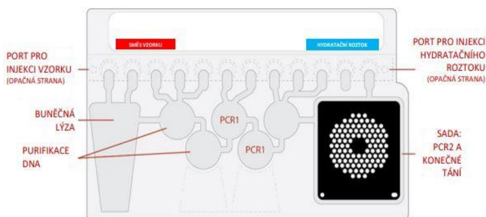
Obrázek 4: Schématické zobrazení FilmArray vaku (zdroj obrázku: www.biofiredx.com )
