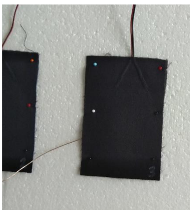
Obrázek 39 Stanovení stupně vyhřívání “pod“ vyhřívací vložkou
