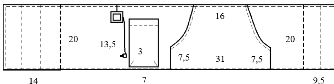
Obrázek 53 Rozměrové parametry pásu
