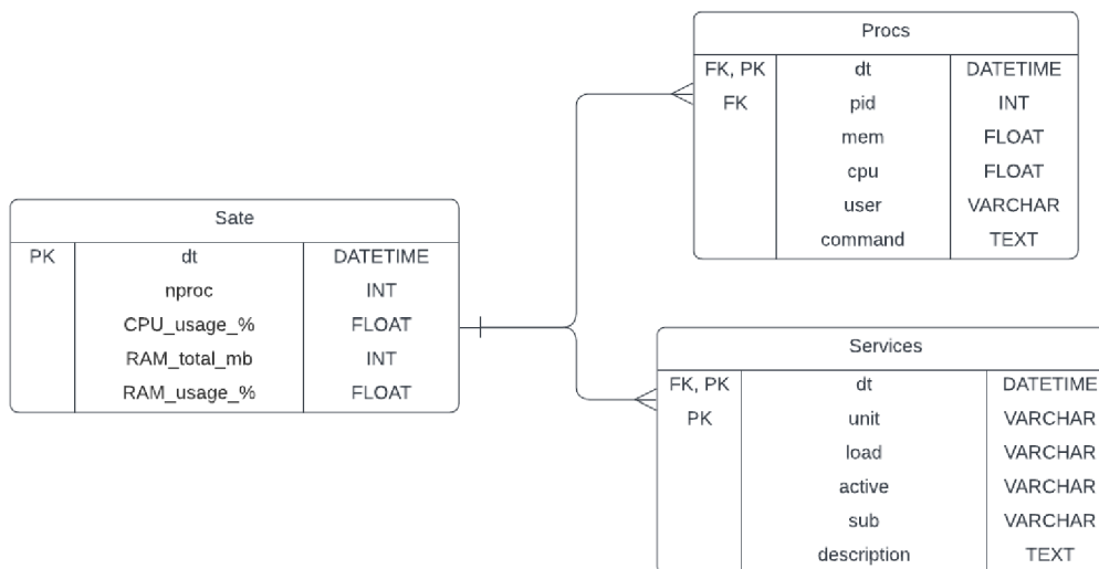
Obrázek 6 – ER diagram ukládání logů (vlastní zpracování)
