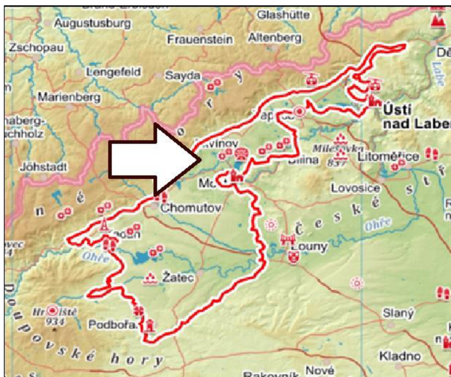
Obr. 5: Mostecká hnědouhelná pánev
