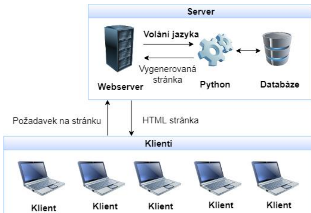
Obr 2.6 Architektura pro webové aplikace [17]
