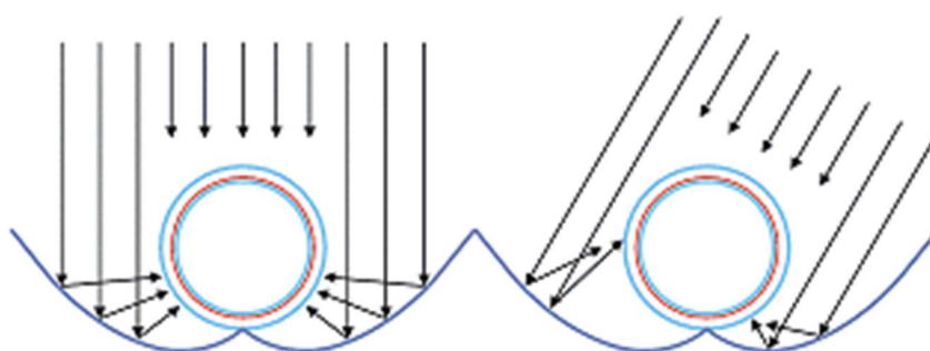
Obrázek 22 Koncentrační solární kolektory pro aplikace v budovách: trubkový Sydney kolektor s reflektorem [4]
