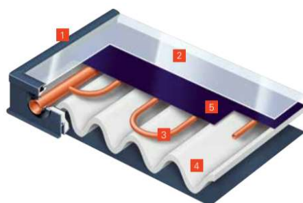
Obrázek 12 Ploché selektivní kolektor [9]
