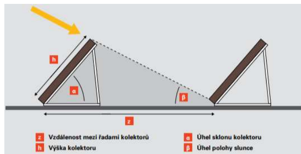
Obrázek 42 Stínění kolektorů [12]
