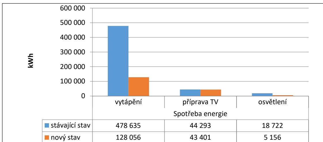
Graf 11 Dodaná energie na spotřebu – porovnání stávajícího a nového stavu
