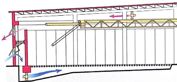
Obrázek č. 1 Schéma průchodu větracího vzduchu a řízení klimatu v boxovém skladu volně ložených brambor Zdroj: Mayer (2014), upraveno autorem
