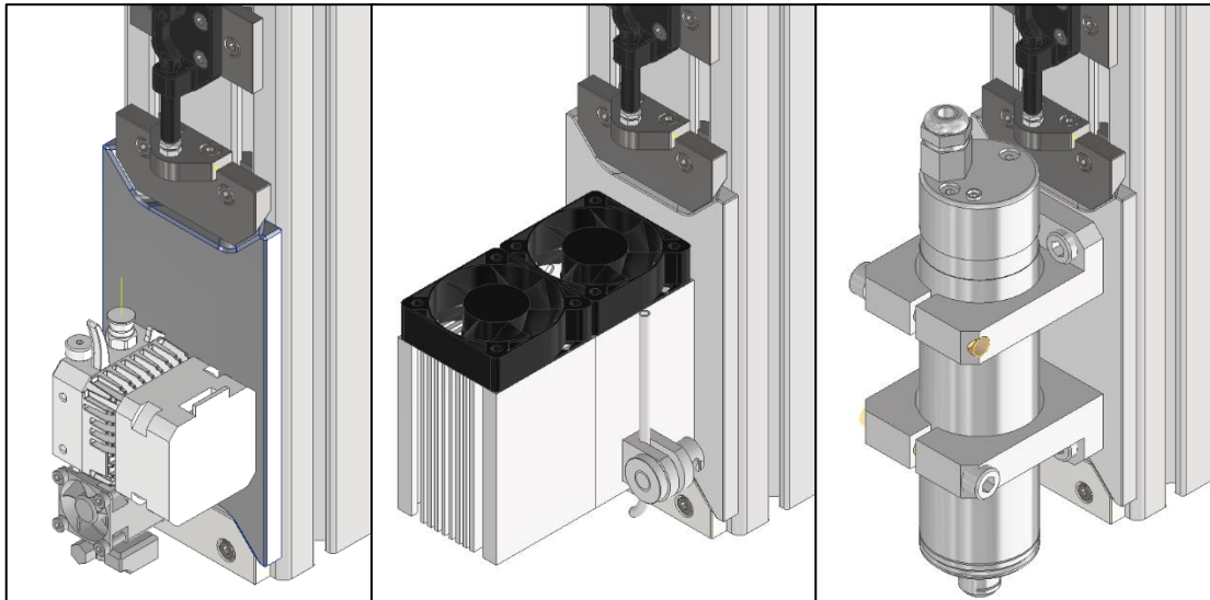
Obrázek 26: Upínání nástrojových periferií
