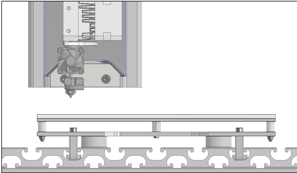
Obrázek 24: Přední pohled – upnutí tiskového stolu
