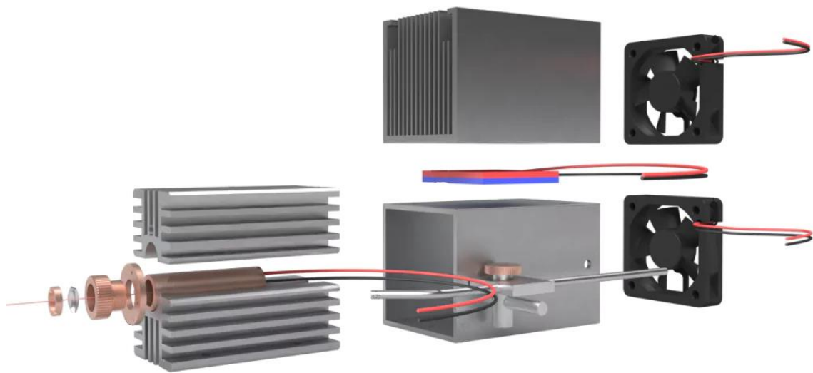
Obrázek 13: Rozložený model laseru [20]
