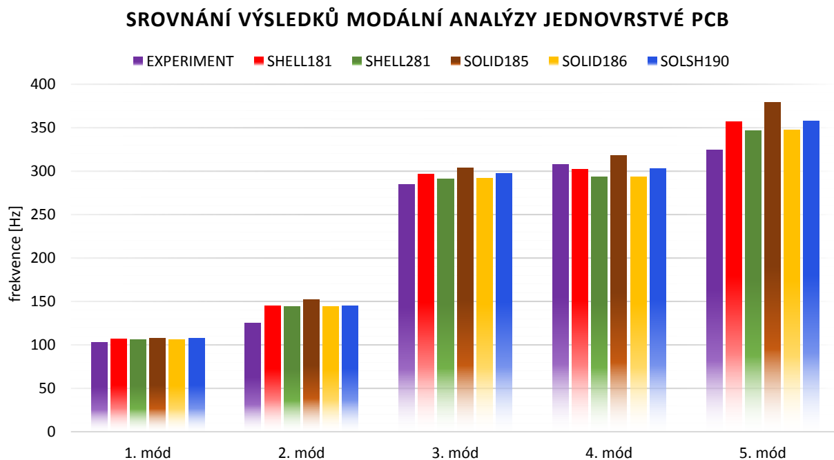
Obr. II-5 Grafické srovnání výsledků modální analýzy jednovrstvé PCB
