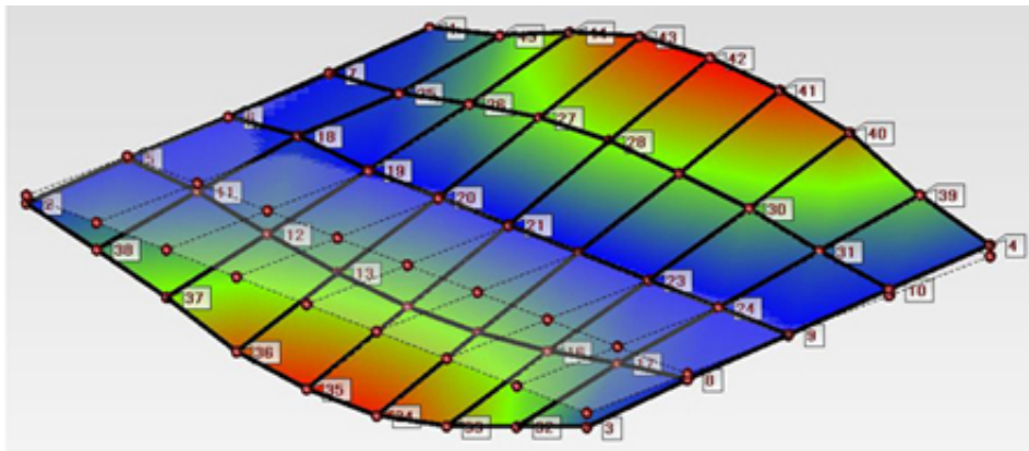
b) 2. vlastní tvar
