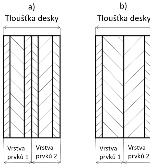
Obr. 8.10 Schematické zobrazení a) chybného nastavení sekci, b) korektního nastavení sekci
