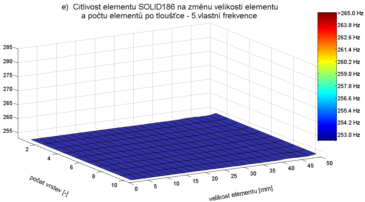
Obr. I-4 Grafické znázornění citlivosti prvku SOLID186 na změnu velikosti hrany a počtu prvků po tloušťce
