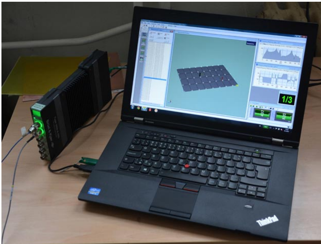
Obr. 9.3 Multianalyzátor PULSE LAN-XI propojený s laptopem. Ve spuštěném softwaru si lze všimnout geometrie desky se zvolenou sítí měřených bodů.
