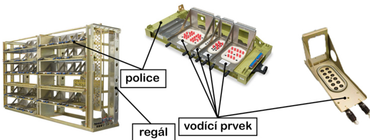
Obr. 6.1 Proky určené k uložení LRU [4]
