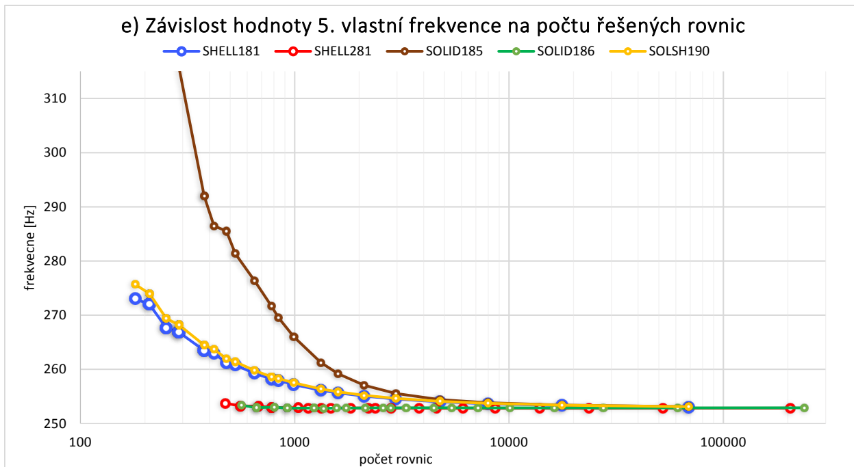
Obr. I-6 Znárodnění závislosti hodnoty vlastní frekvence na počtu řešených rovnic u jednotlivých prvků
