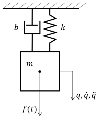
Obr. 6.7 Systém s jedním stupněm volnosti – hmotnosti m , tuhost k , tlumení b , budicí síla f(t) , posuv q , rychlost \dot{q} a zrychlení \ddot{q} .
