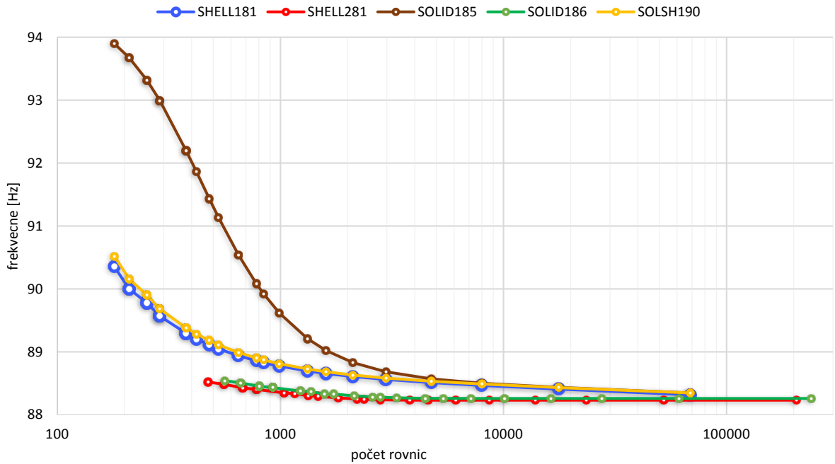
a) Závislost hodnoty 1. vlastní frekvence na počtu řešených rovnic
