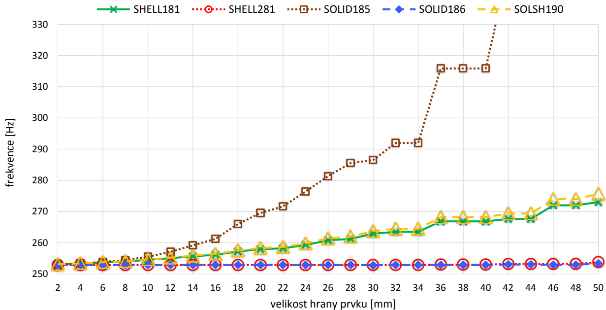
Obr. I-2 Srovnání citlivosti použitých elementů na změnu velikosti hrany
