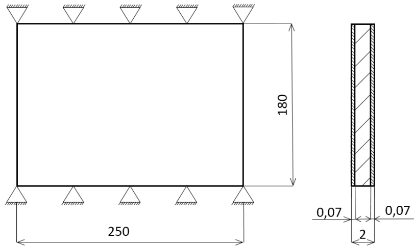
Obr. 8.8 Schematický náčrt geometrických rozměrů vícevrstvé PCB
