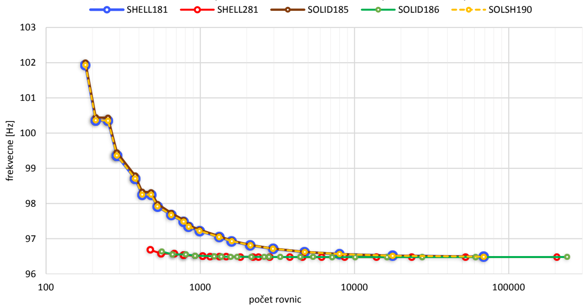
b) Závislost hodnoty 2. vlastní frekvence na počtu řešených rovnic
