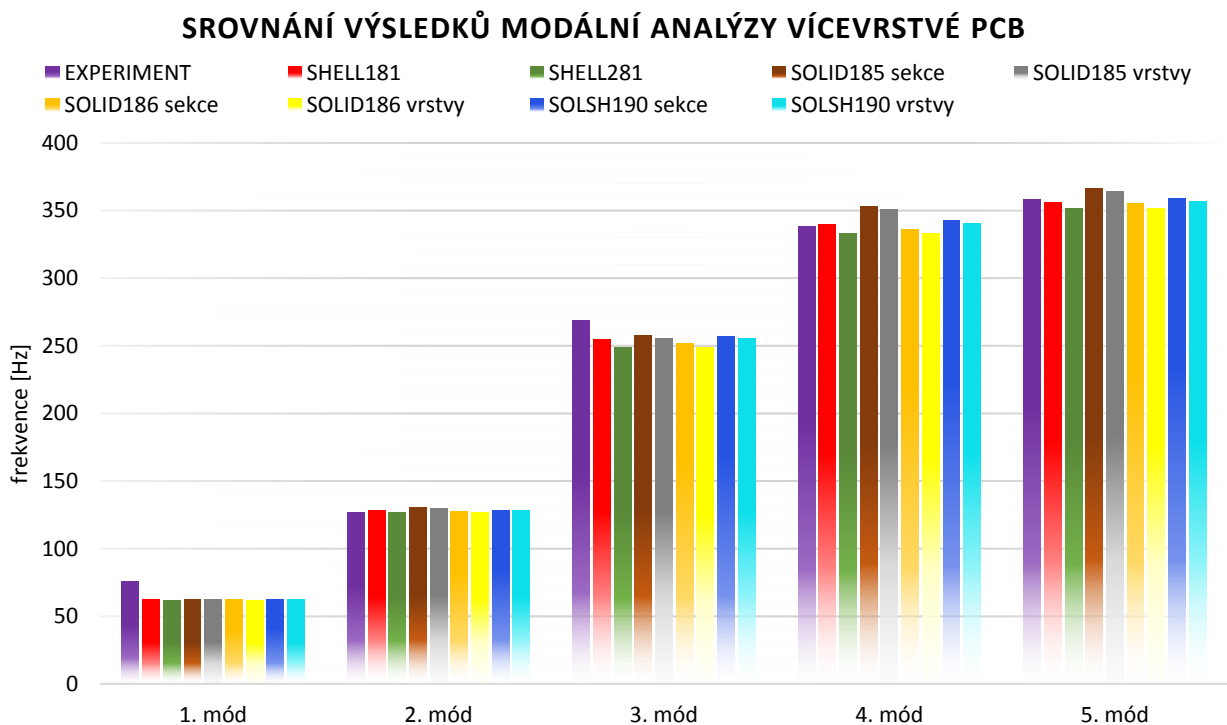
Obr. 10.2 Grafické porovnání výsledků modální analýzy vícevrstvé desky, stanovené výpočtovým a experimentálním modelováním
