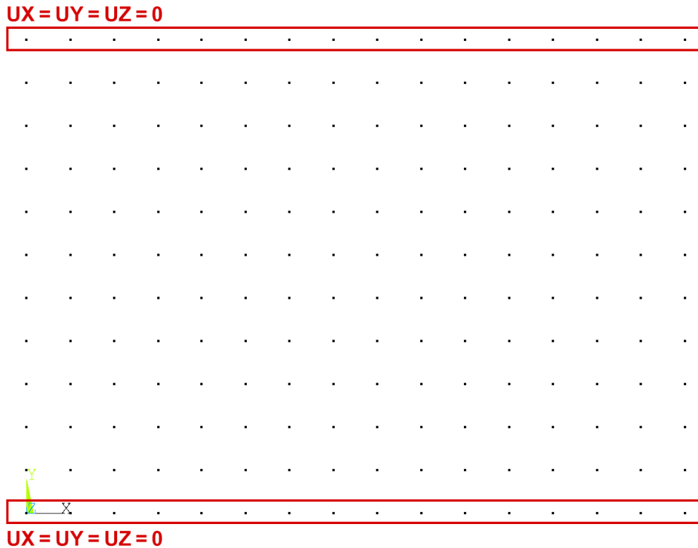
Obr. 8.3 Zobrazen uzlov body s vyznaenm mstem aplikace okrajovch podmnek
