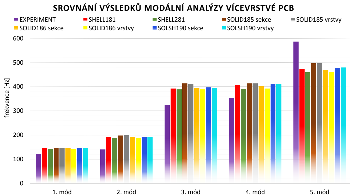
Obr. II-6 Grafické srovnání výsledků modální analýzy vícevrstvé PCB
