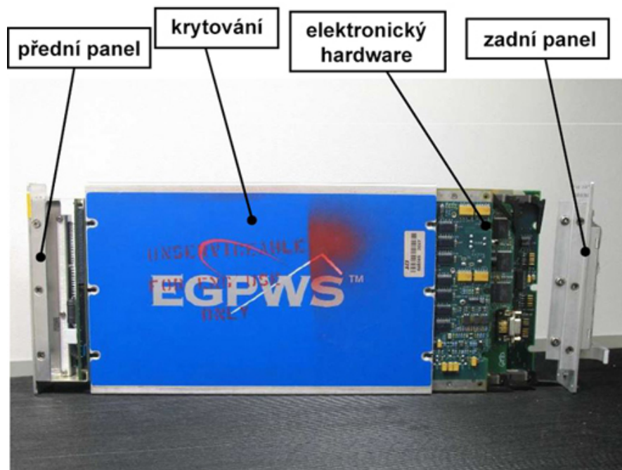
Obr. 6.4 Pohled na jednotlivé části jednotky LRU [5]
