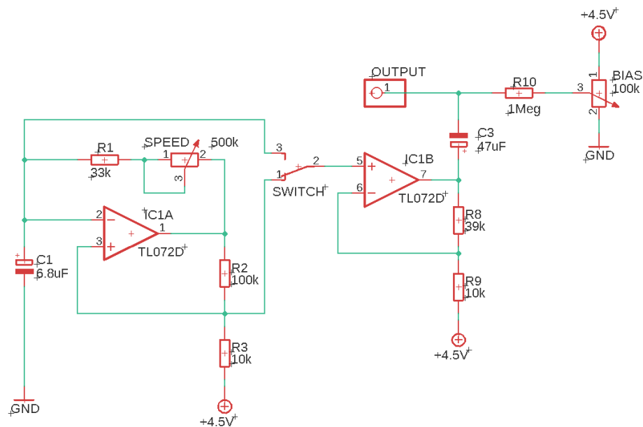
obr. 3.12 Relaxační oscilátor s průběhy obdélník, trojúhelník
