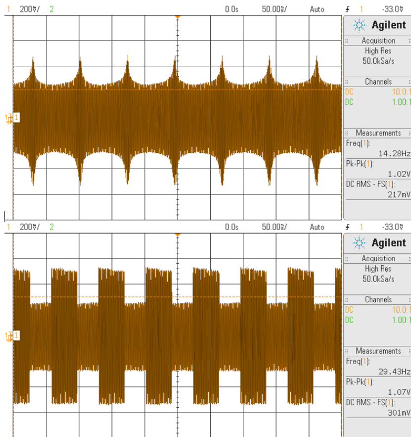
obr. 6.11 Měření obvodu tremolo (střední hloubka modulace)
