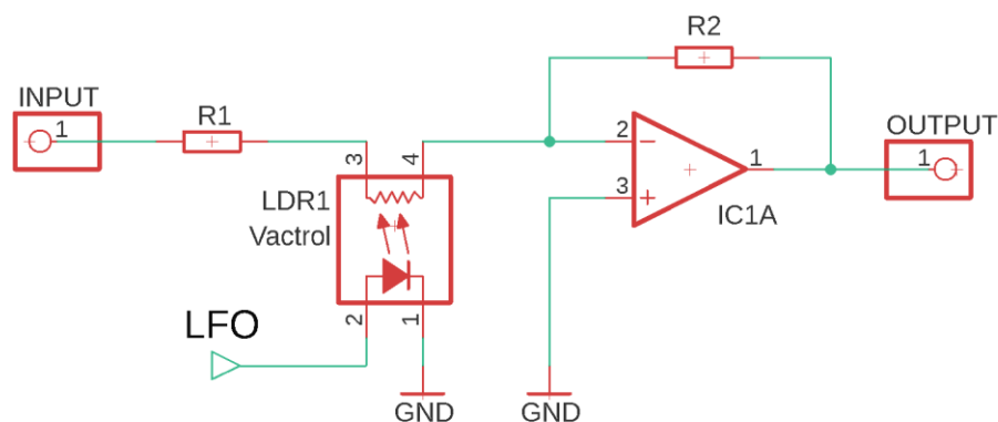
obr. 3.10 Základní obvod VCA s optočlenem
