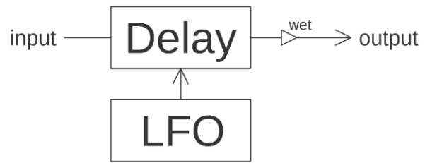
obr. 1.5 Jednoduché Vibrato se zpoždřovacím členem
