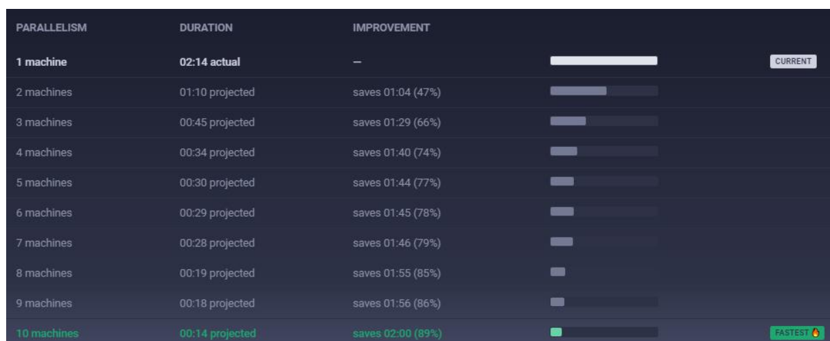
Obrázek 19 – Výsledek automatického testování, práce autora
