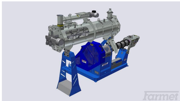
Obrázek 13: Kondicionér FK 500 v instalaci se extrudérem FE 500 od společnosti FARMET a.s. [42]
