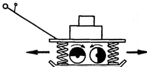
Obr. 21 Vibrační deska s oboustranným pohybem [50]
