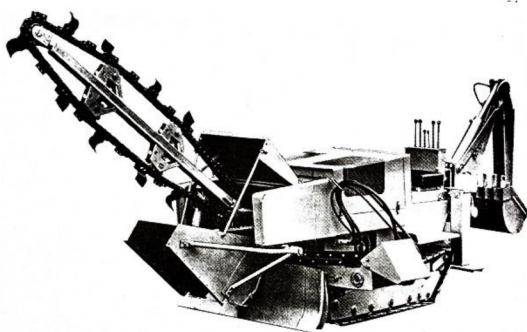
Obr. 11 Řetězový rýhovač [25]
