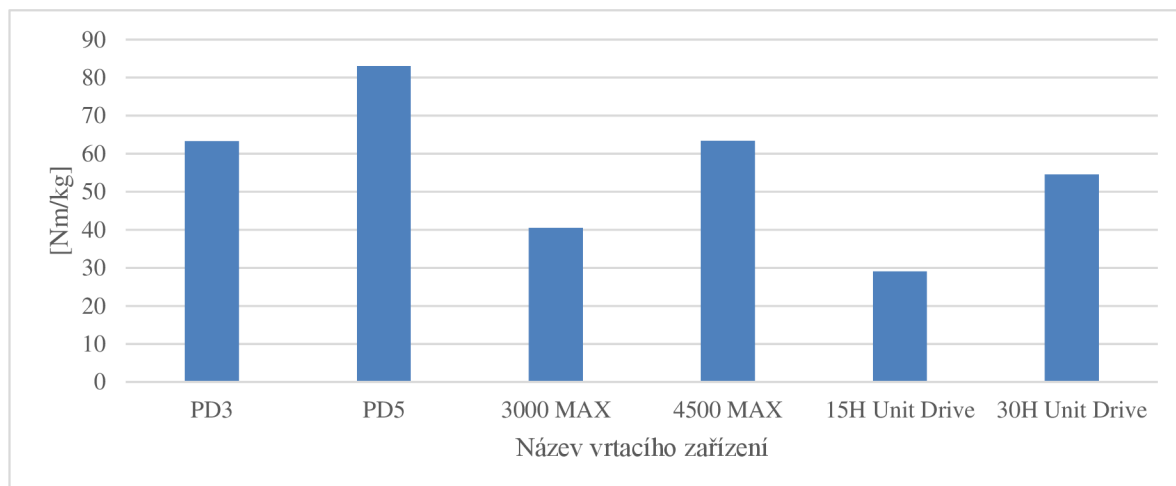
Obr. 9 Graf poměru maximálně dosažitelného kroučícího momentu ke hmotnosti hydromotoru
