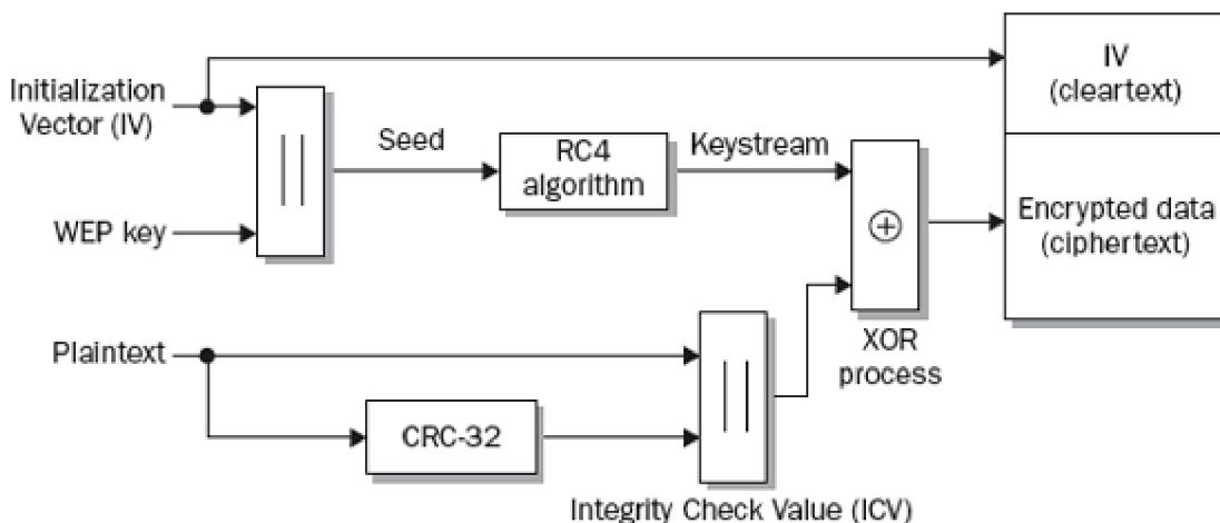
Obrázek 2.1: Průběh šifrování dat u zabezpečení WEP 1
