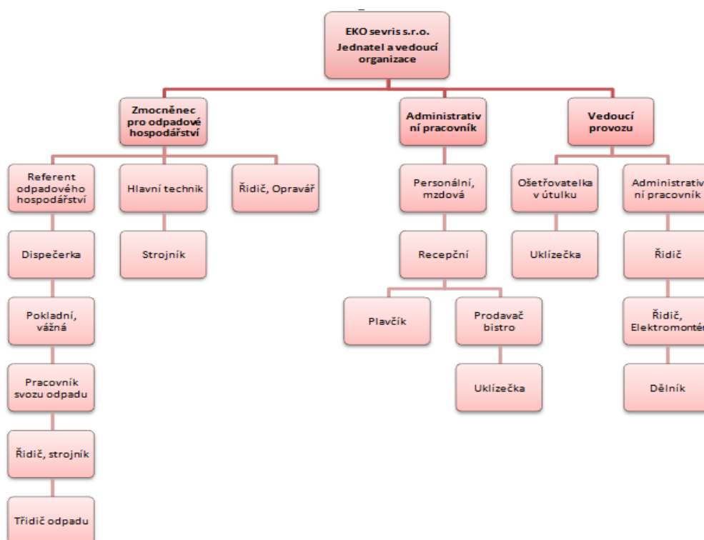
Obr. 2.1 Organizační struktura
