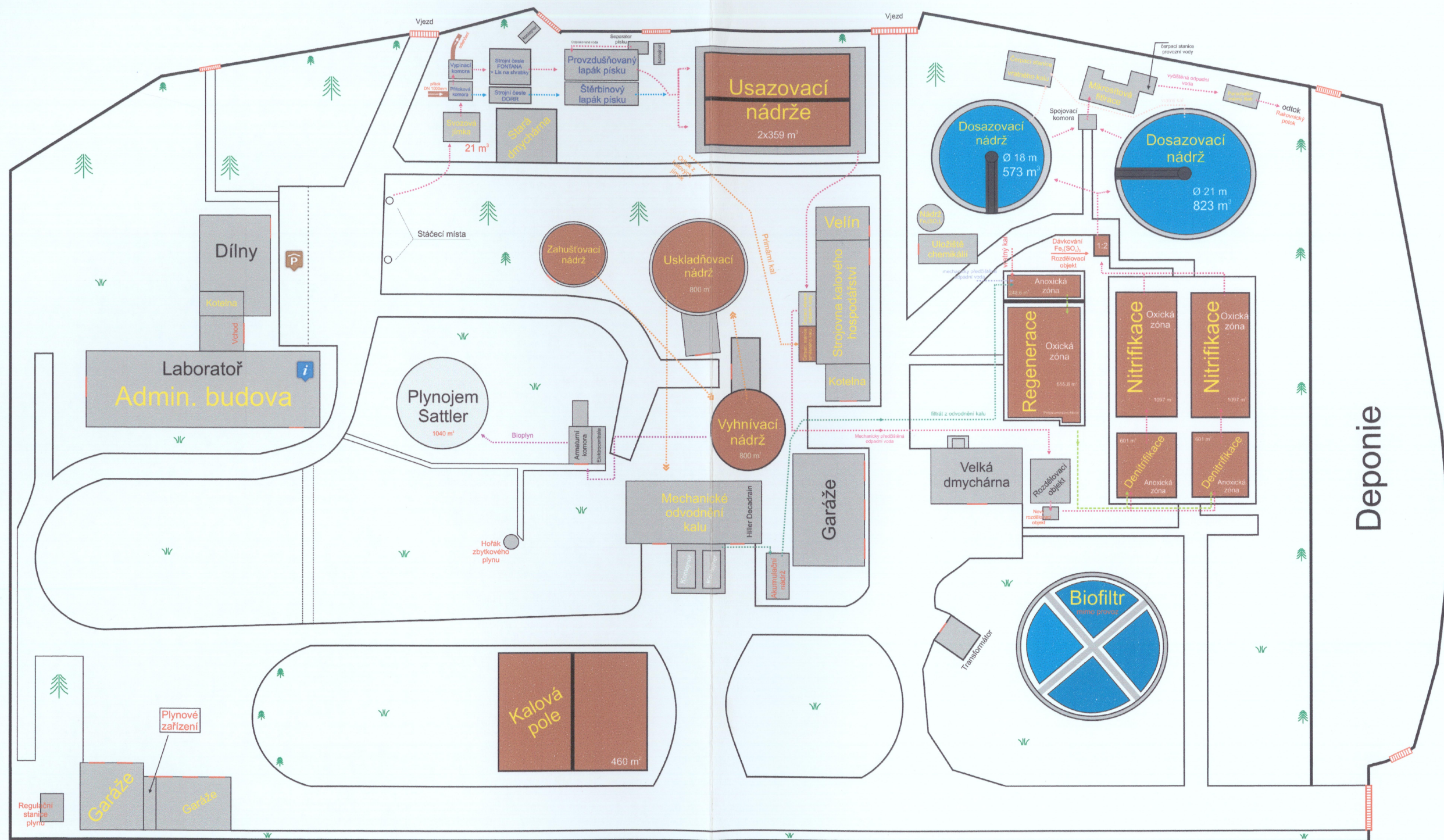
Příloha č. 5: Situace čistírny odpadních vod Rakovník 2014
