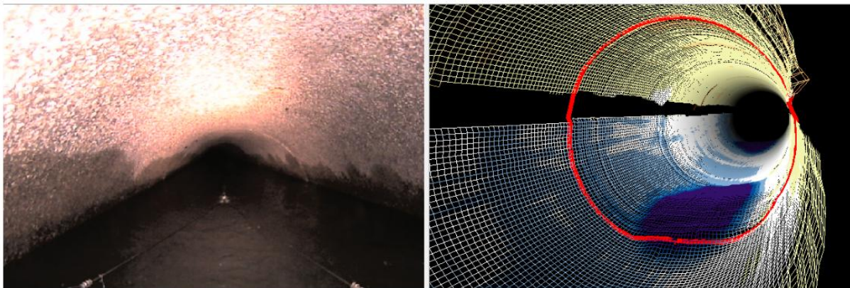
Obr. 9.6 Příklad vizuální kontroly pomocí plovákového sonaru a následné výsledky inspekce [26]
