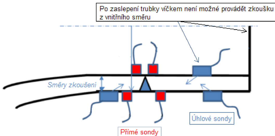
Obr. 46 Nákres podmínek zkoušky ultrazvukem u svaru č. 4.
