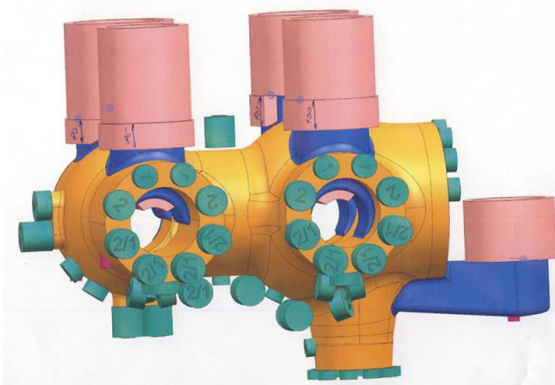
Obr. 29 Simulace lití bloku regulačního ventilu v Magma.
