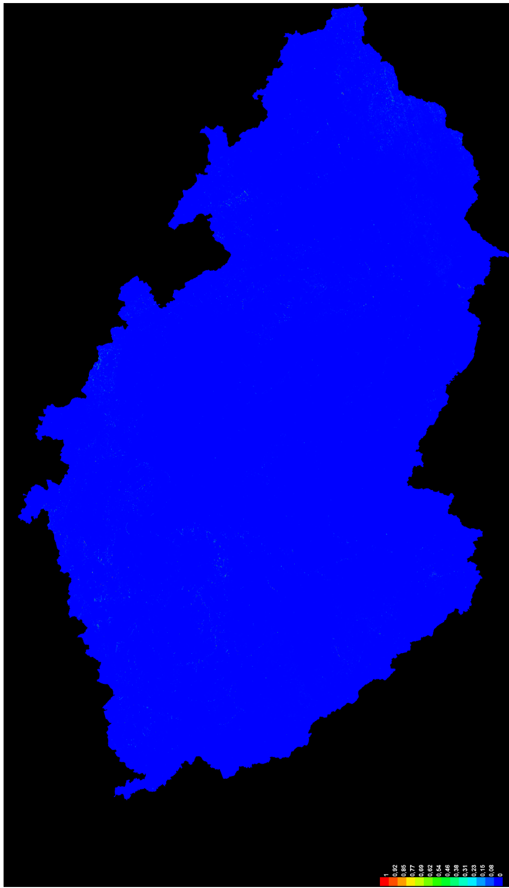
Obrázek 6. Habitatový model jasoně červenookého na Slovensku. Odstíny modré představují méně vhodná místa, odstíny zelené podmínky, ve kterých se jasoně červenooký běžně vyskytuje, odstíny červené lokalizují obzvláště vhodné podmínky prostředí pro výskyt druhu.
