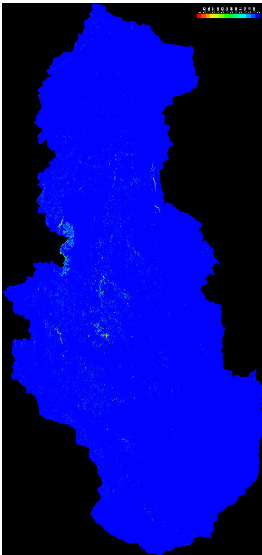
Obrázek 1. Habitatový model jasoné červenookého na Slovensku. Odstíny modré představují méně vhodná místa, odstíny zelené podmínky, ve kterých se jason běžné vyskytuje, odstíny červené lokalizují obzvláště vhodné podmínky prostředí pro výskyt druhu.
