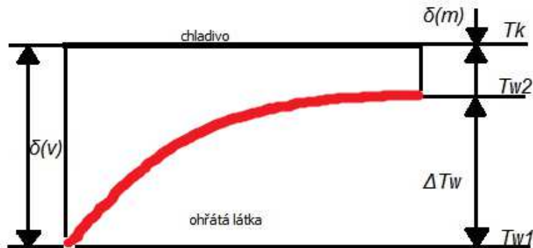
Obr. 8 – Průběh teplot v kondenzátoru (srážníku)
