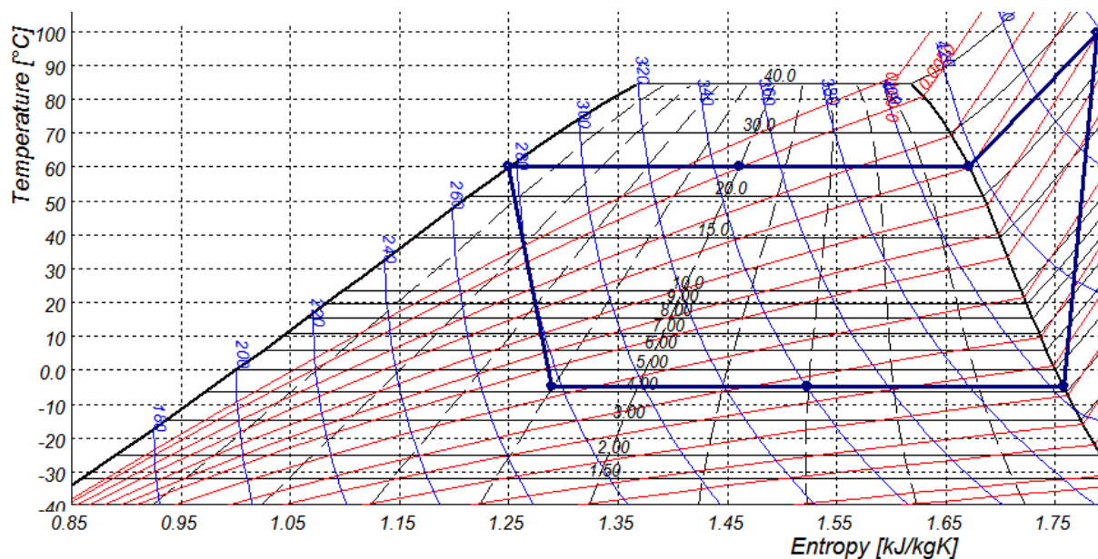
Obr. 25 – Zobrazení funkce tepelného čerpadla v T-s diagramu. (Zdroj: Solkane)
