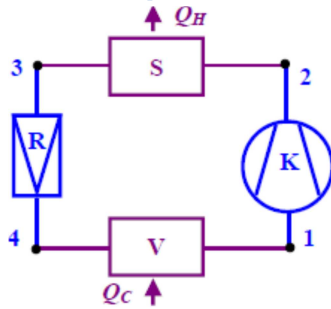
Obr. 5 – Schéma tepelného čerpadla [10]
