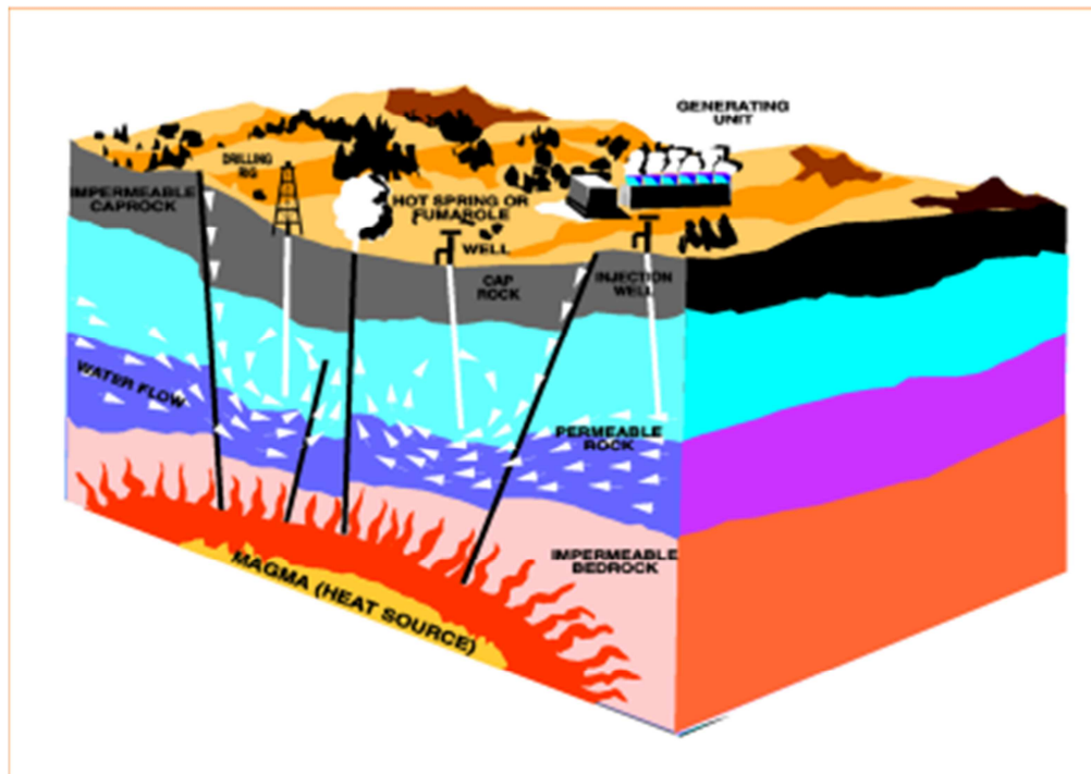
Obr. 17 – Obecně znázorněná struktura profilu Země [16]
