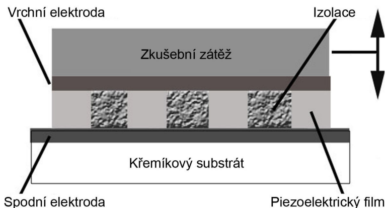
Obr. 3 – Piezoelektrický akcelerometr [1]
