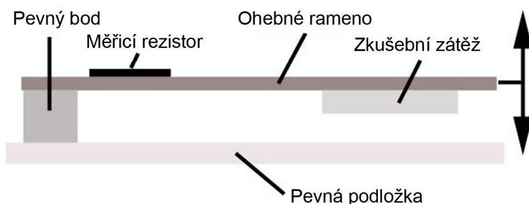
Obr. 2 – Tenzometrický akcelerometr [1]
