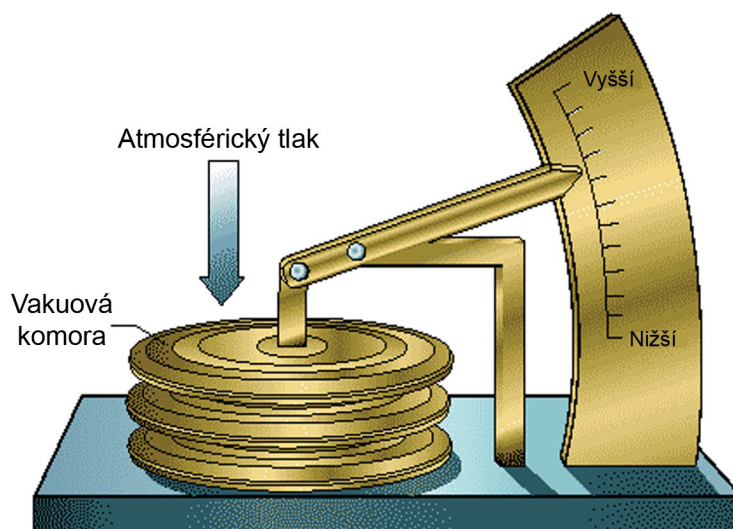
Obr. 6 – Princip aneroidu [4]
